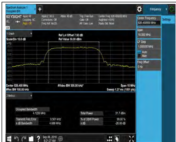
WCDMA Band V_4132
