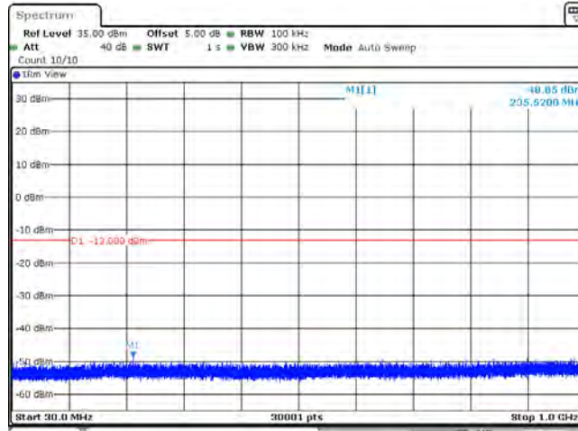
Band4_20MHz_QPSK_20175_1RB#0
