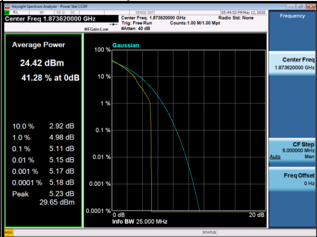
16QAM-26140
