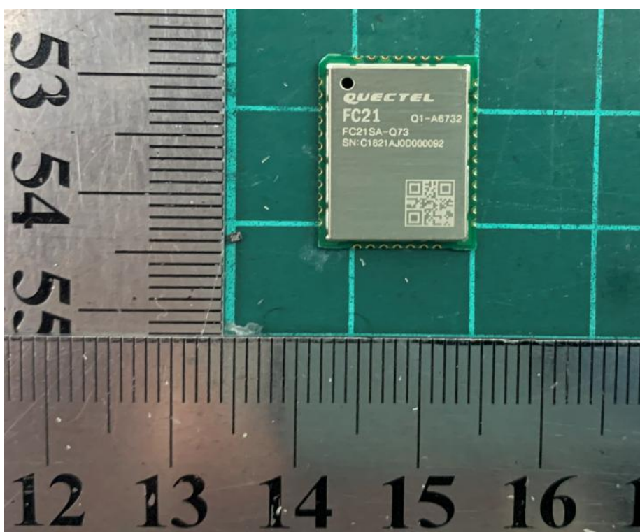
a: EUT
