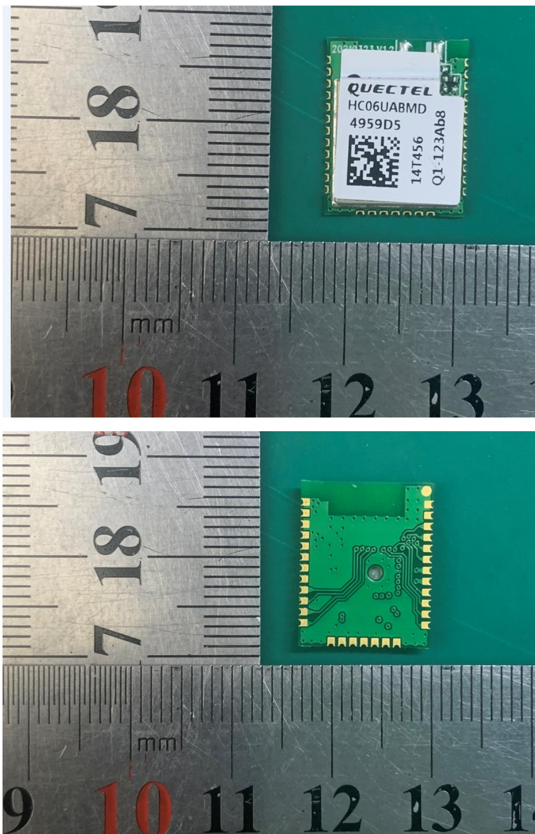
a: EUT
