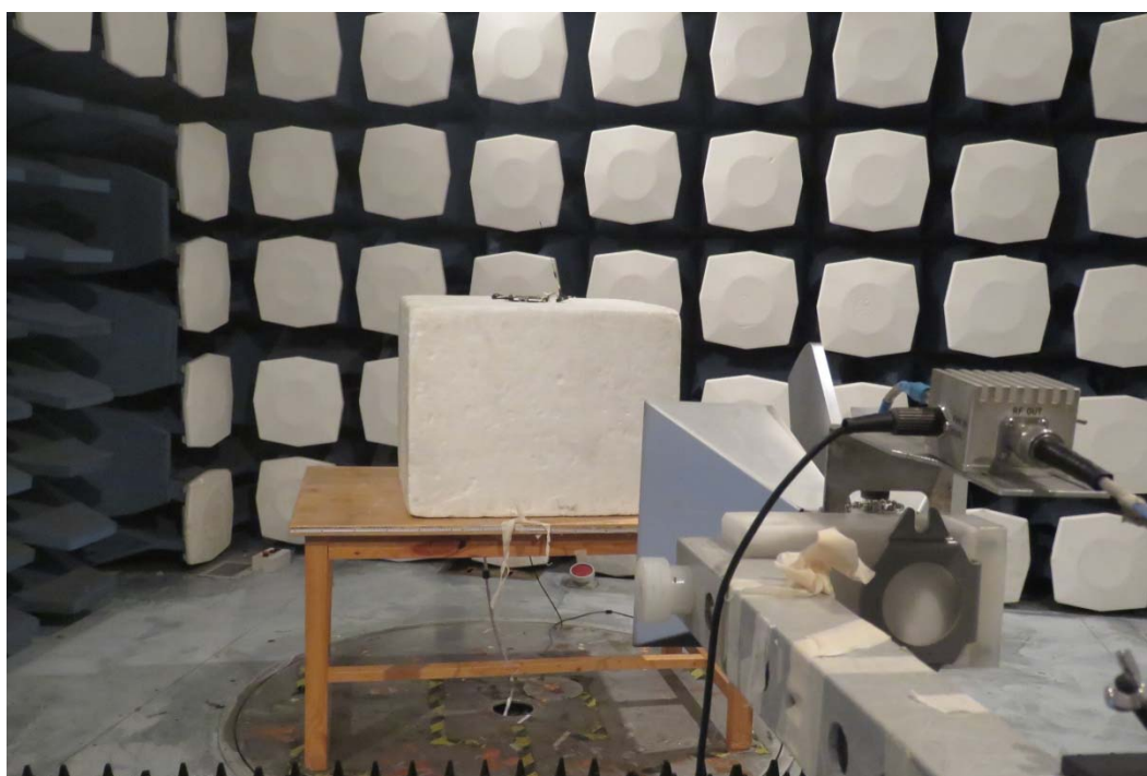
1GHz-18GHz
