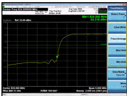
LTE Band 5 QPSK 1.4MHz CH-Low 1RB
