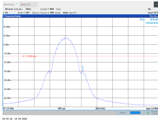
GSM1900-810
