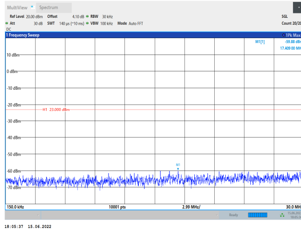
GSM1900-512-0.15~30MHz
