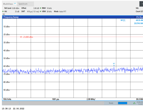
Band71-20MHz-QPSK-133222-1RB#0-Range2:0.15~30MHz
