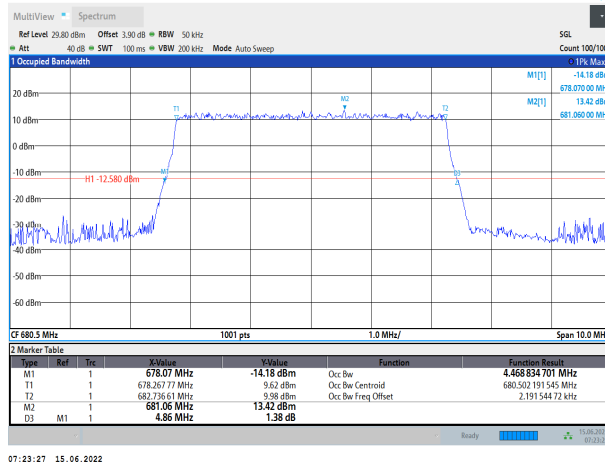
Band71-5MHz-QPSK-133297-25RB#0
