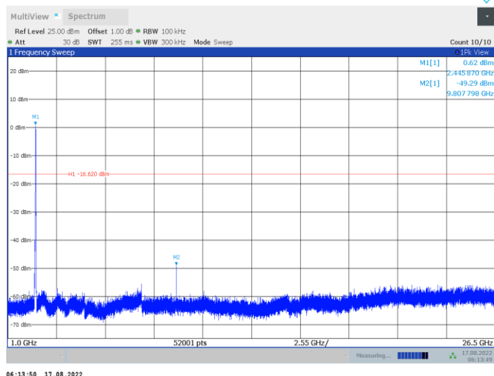
11n40MIMO Ant2 2452 1000~26500
