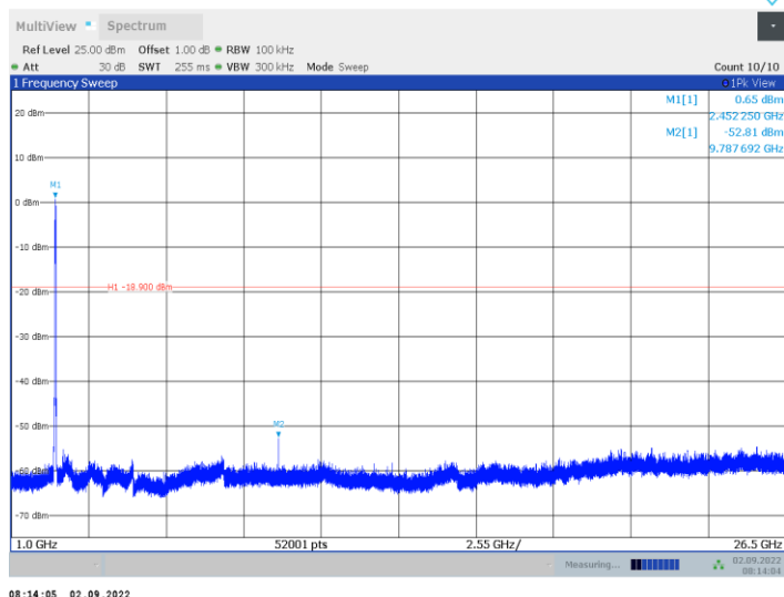
11n40MIMO Ant2 2447 1000~26500
