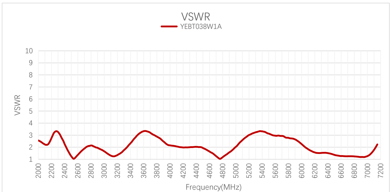
VSWR
