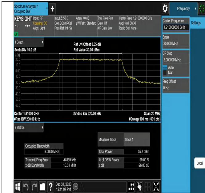
Band25-10MHz-QPSK-26640-50RB#0-PASS
