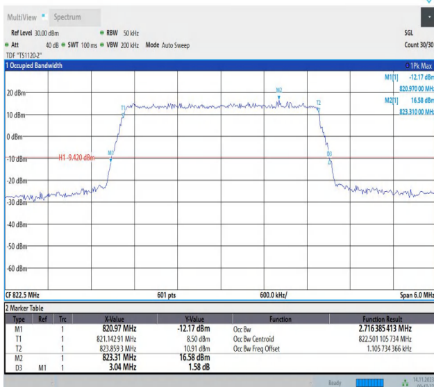
26(814-824)-3MHz-QPSK-26775-15RB#0-PASS
