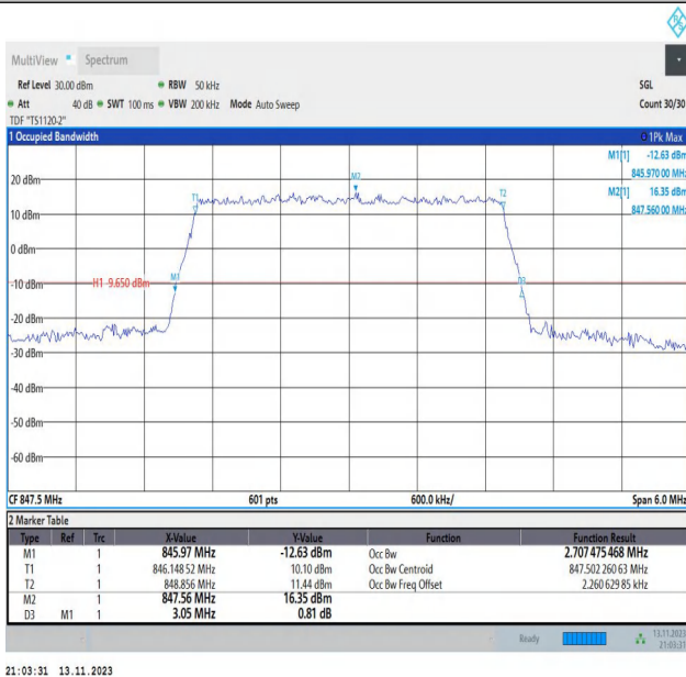
26(824-849)-3MHz-QPSK-27025-15RB#0-PASS
