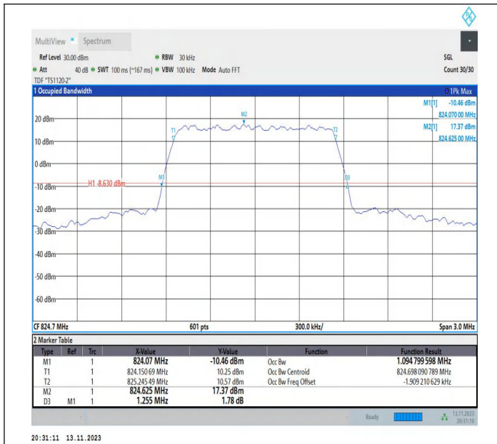
26(824-849)-1.4MHz-QPSK-26797-6RB#0-PASS
