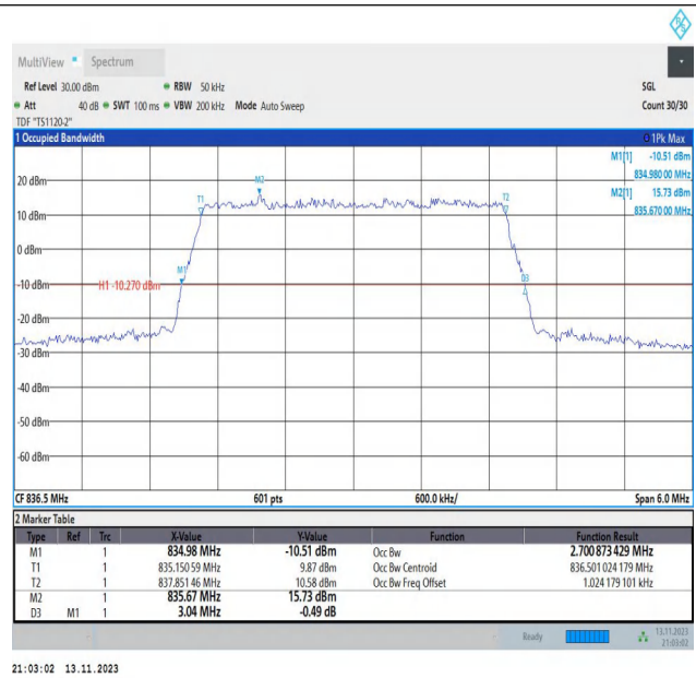
26(824-849)-3MHz-16QAM-26915-15RB#0-PASS
