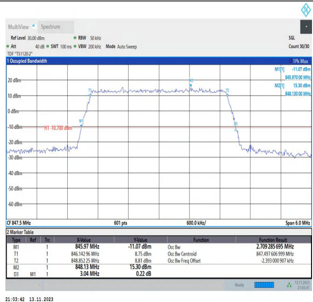
26(824-849)-3MHz-16QAM-27025-15RB#0-PASS
