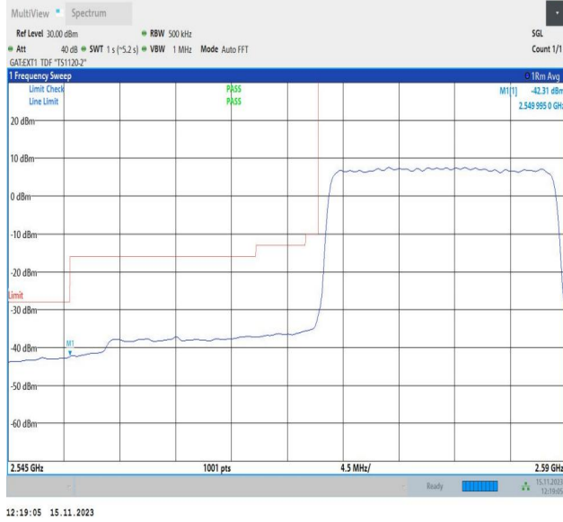
Band38_20MHz_QPSK_37850_100RB#0
