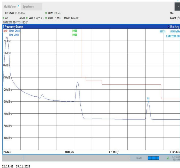
Band38_20MHz_QPSK_38150_1RB#0
