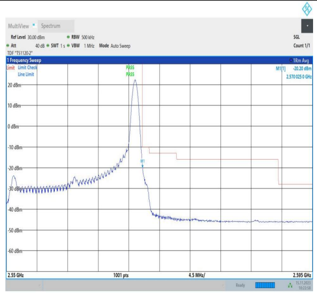
Band7_20MHz_16QAM_21350_1RB#99
