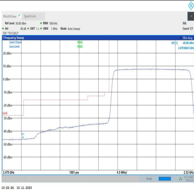
Band7_20MHz_QPSK_20850_100RB#0
