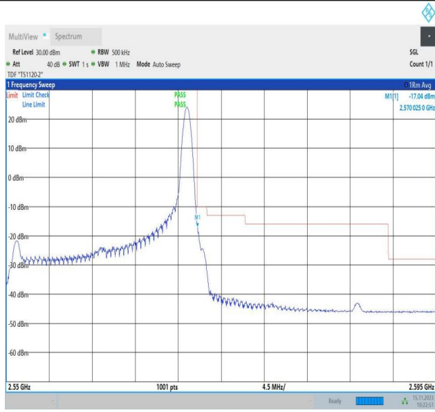
Band7_20MHz_QPSK_21350_1RB#99
