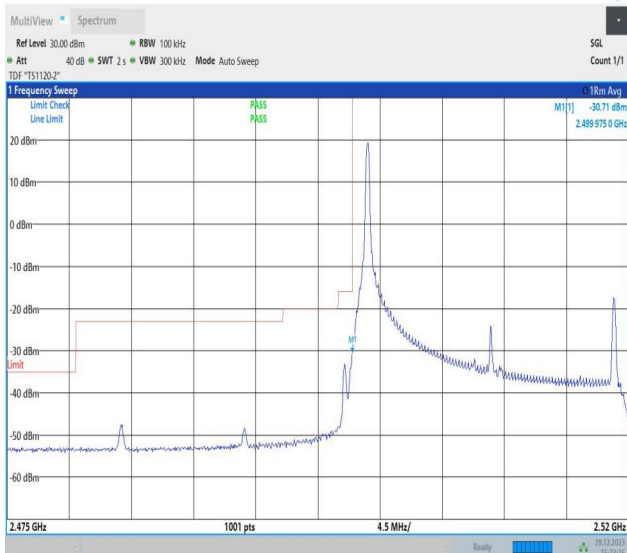
Band7_20MHz_64QAM_20850_1RB#0
