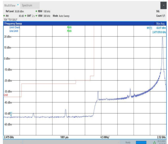
Band7_20MHz_64QAM_20850_1RB#99
