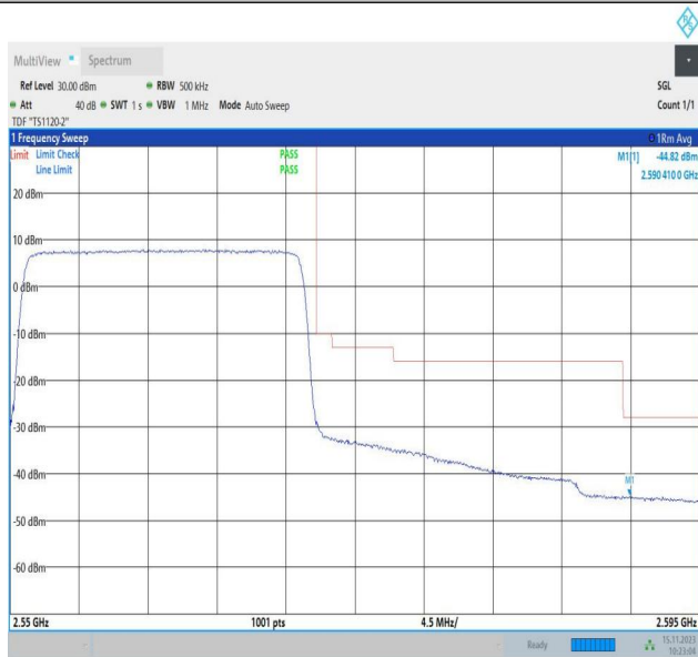
Band7_20MHz_QPSK_21350_1RB#99
