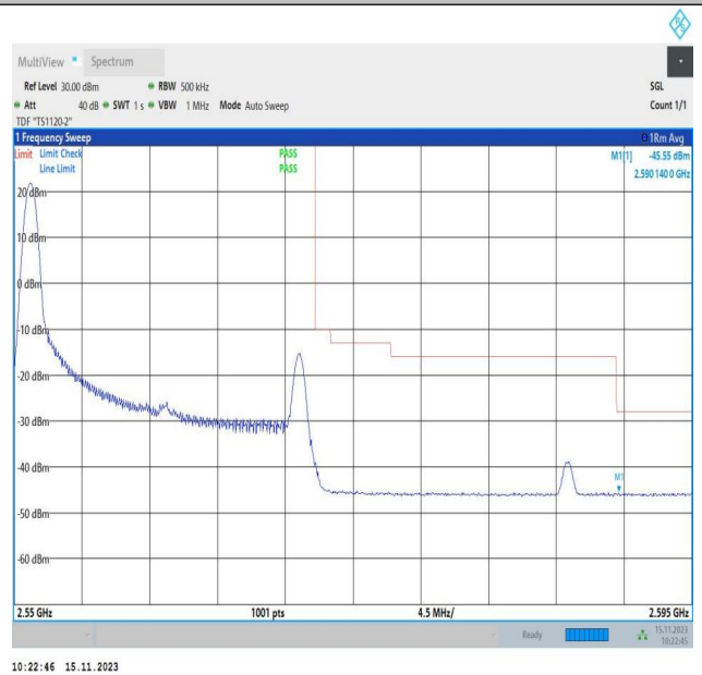
Band7_20MHz_16QAM_21350_1RB#0
