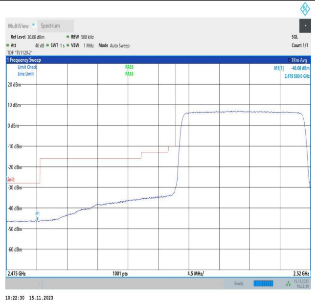
Band7_20MHz_16QAM_20850_100RB#0
