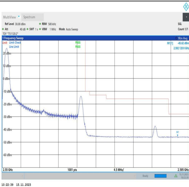
Band7_20MHz_QPSK_21350_1RB#0
