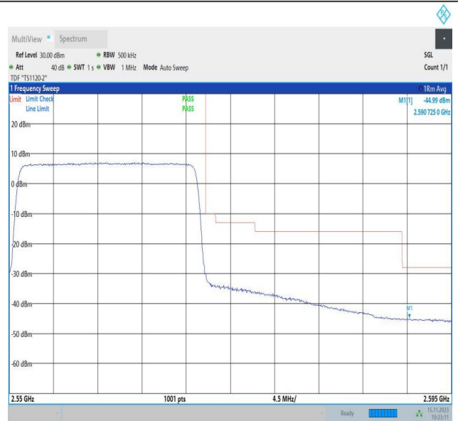
Band7_20MHz_16QAM_21350_1RB#99
