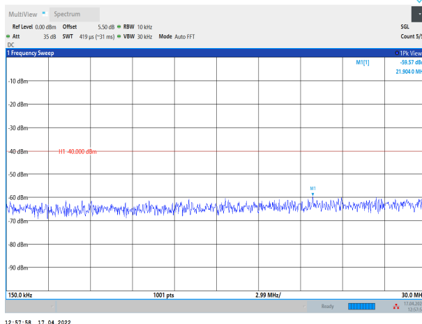
Band30-10MHz-QPSK-27710-1RB#0-Range2:0.15~30MHz
