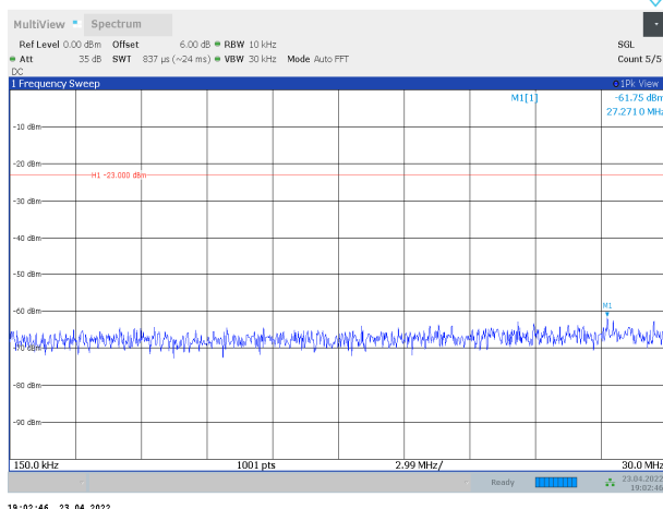
Band42-20MHz-QPSK-42190-1RB#0-Range2:0.15~30MHz
