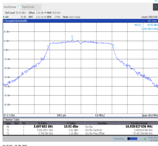
11a-Ant1-5700
