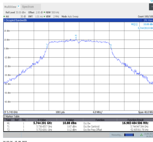
11a-Ant1-5745
