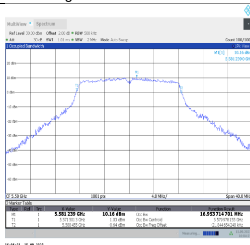
11a-Ant1-5580
