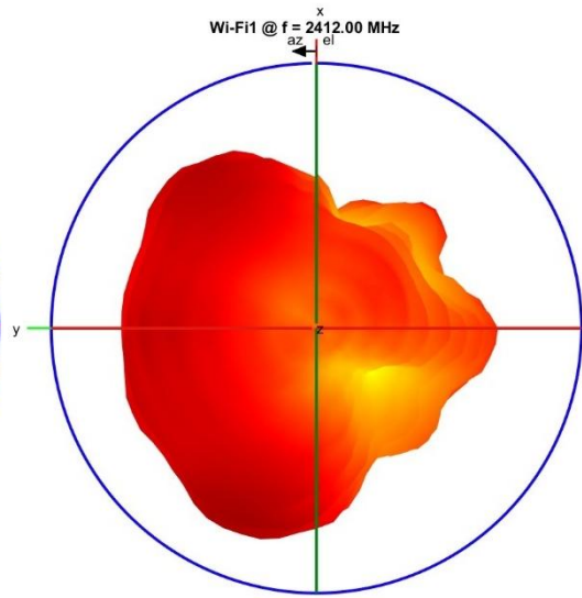
Wi-Fi1
