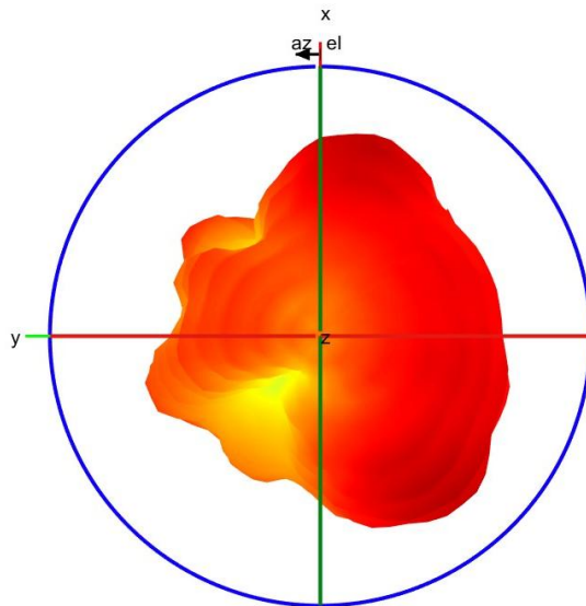
Wi-Fi0/BT
