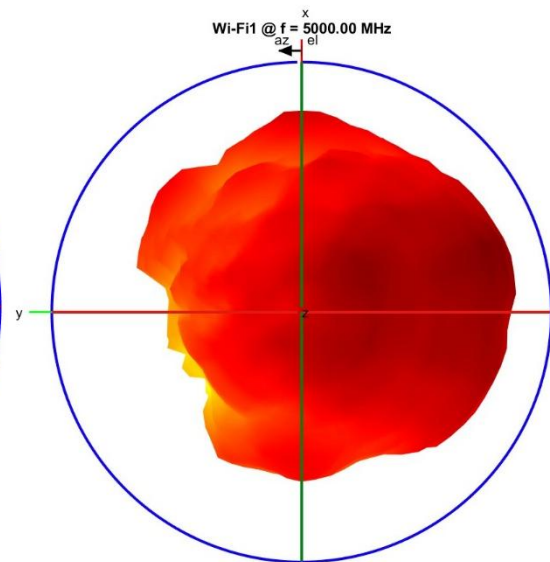
Wi-Fi1
