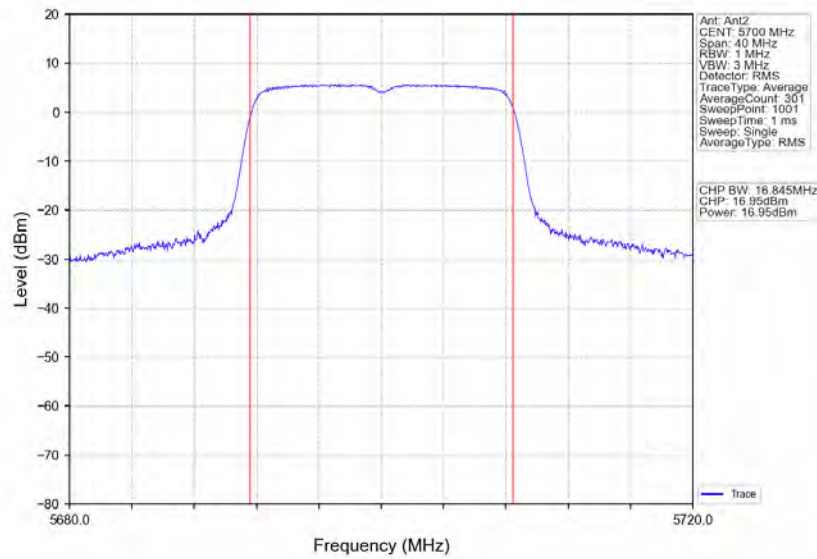
802.11a HCH 5700MHz Ant2 NTVN
