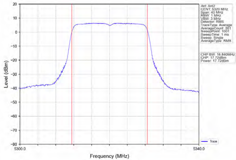
802.11a HCH 5320MHz Ant2 NTNv
