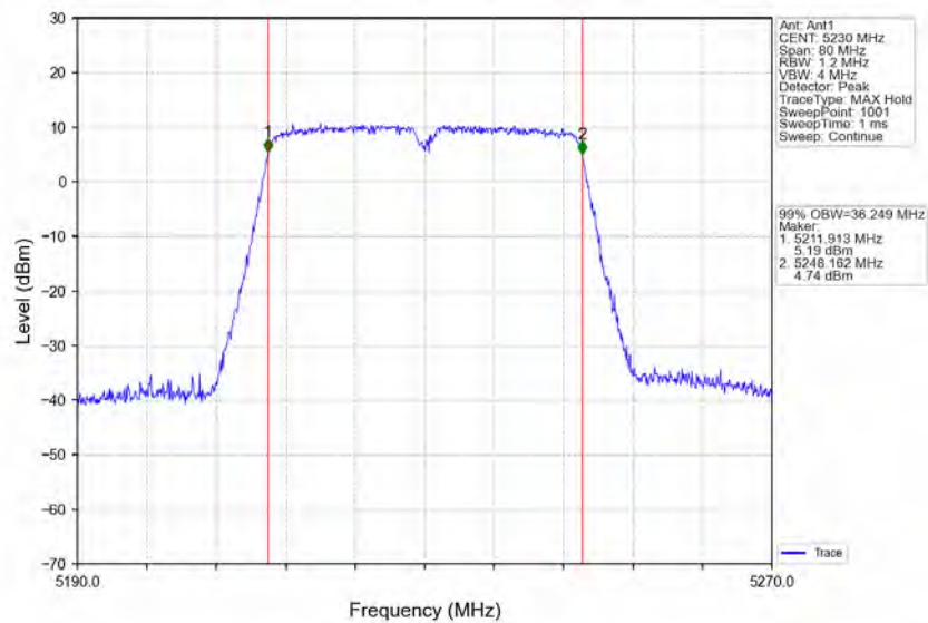
802.11n(HT40)_HCH_5230MHz_Ant1_NTN
