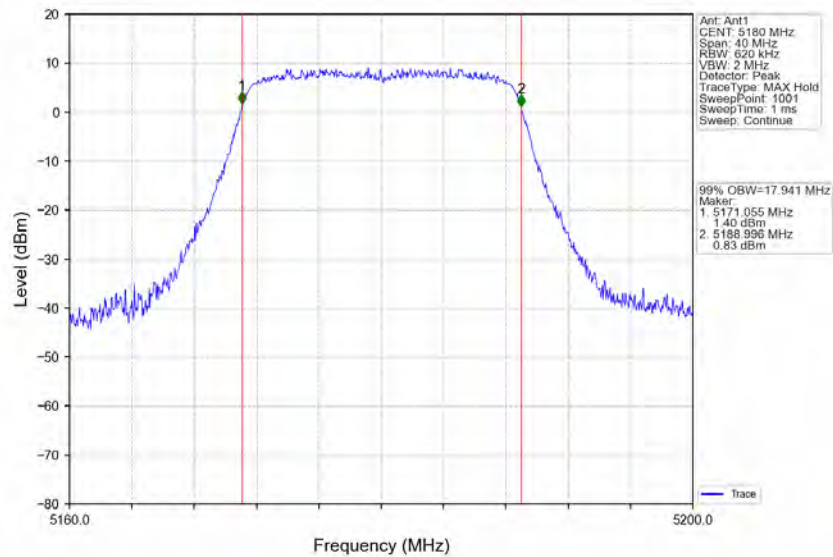
802.11n(HT20)_LCH_5180MHz_Ant1_NTN
