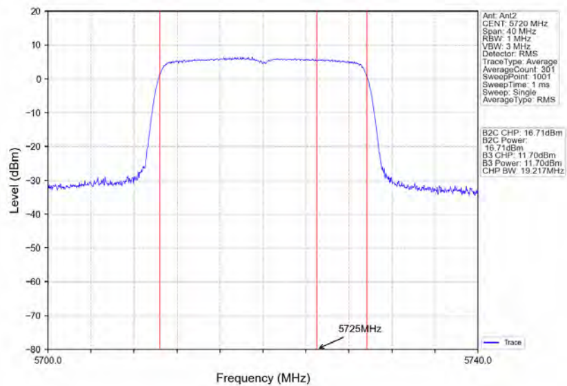
802.11ax(HEW20) HCH 5720MHz RU242 Left Ant2 NTN
