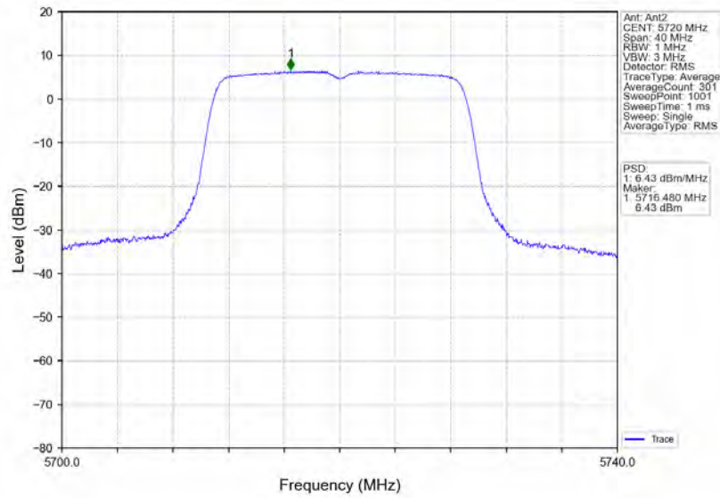
802.11n(HT20) HCH 5720MHz MIMO NTN
