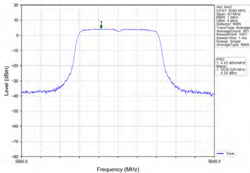
802.11a_MCH_5580MHz_Ant2_NTNV
