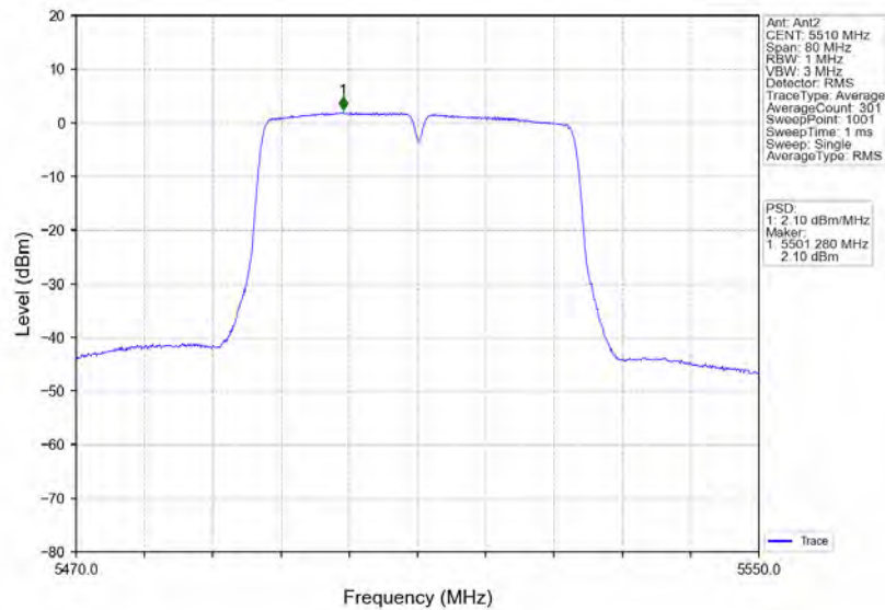
802.11n(HT40) LCH 5510MHz Ant2 NTN
