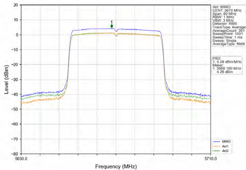
802.11ax(HEW40) HCH 5670MHz RU484 Left MIMO NTN
