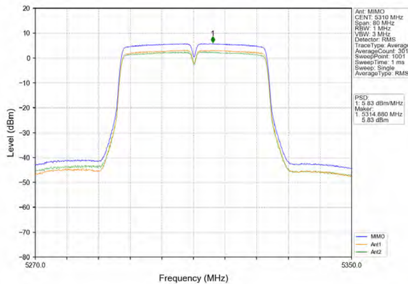
802.11n(HT40) HCH 5310MHz MIMO NTVN
