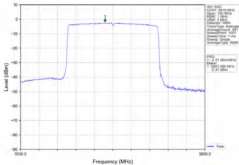
802.11ax(HEW80) HCH 5610MHz RU996 Left Ant2 NTN
