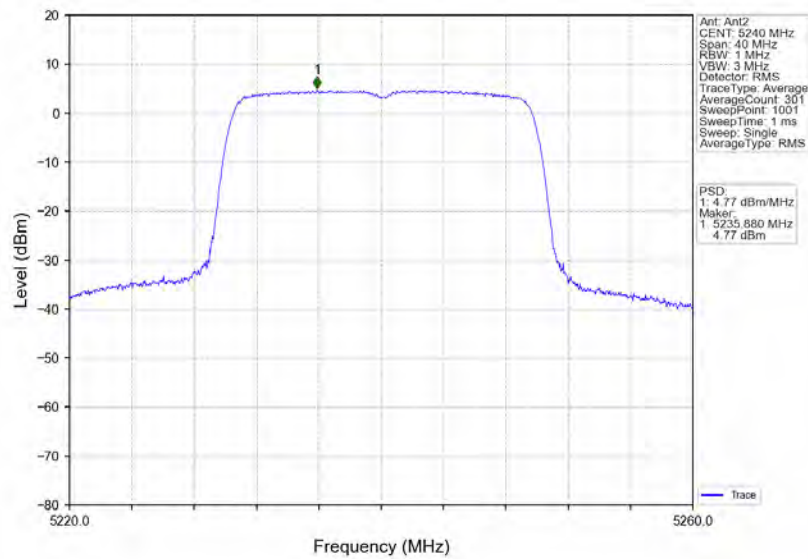
802.11ax(HEW20) HCH 5240MHz RU242 Left MIMO NTN
