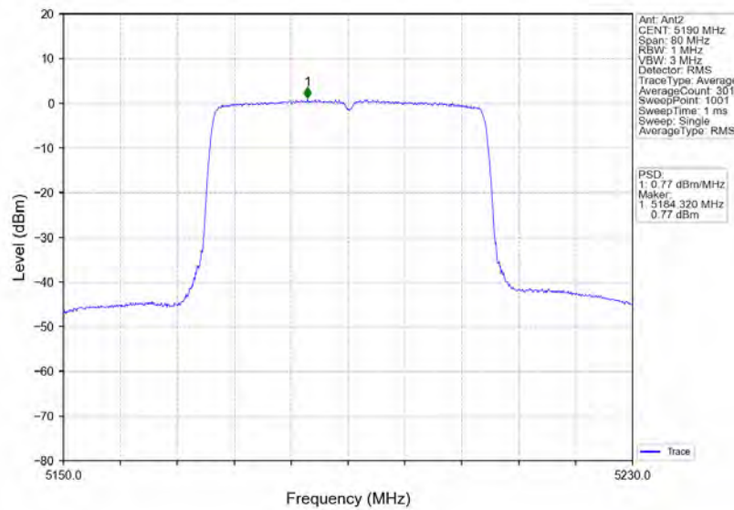
802.11ax(HEW40) LCH 5190MHz RU484 Left MIMO NTN
