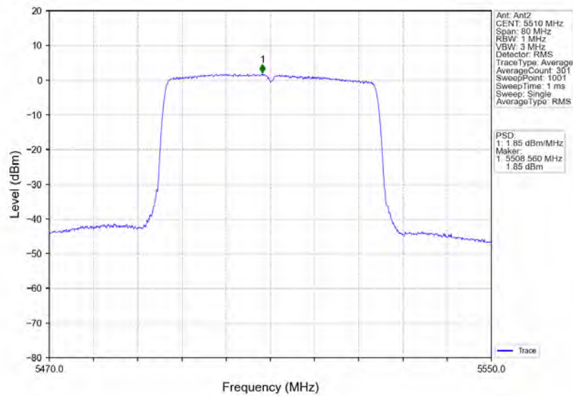
802.11ax(HEW40) LCH 5510MHz RU484 Left MIMO NTN
