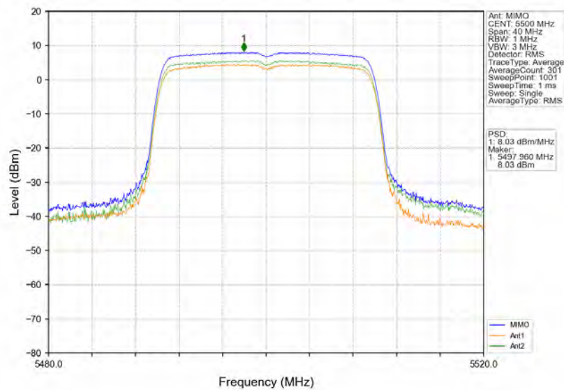
802.11ax(HEW20) LCH 5500MHz RU242 Left MIMO NTN
