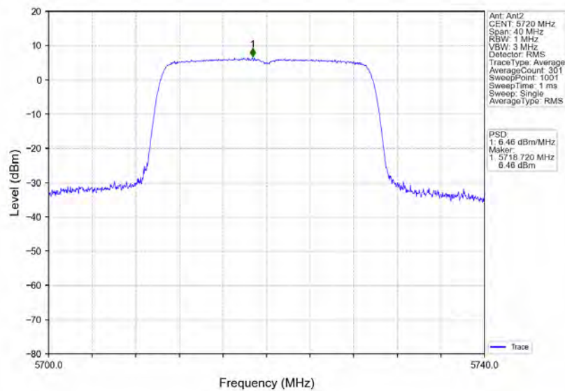
802.11ax(HEW20) HCH 5720MHz RU242 Left Ant2 NTN
