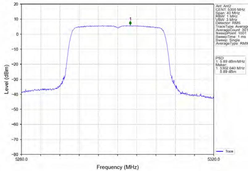
802.11ax(HEW20) MCH 5300MHz RU242 Left MIMO NTN
