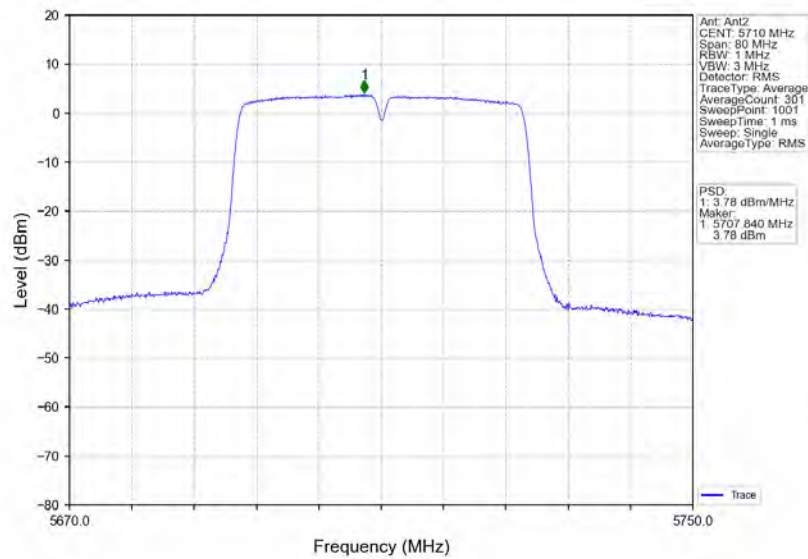
802.11n(HT40) HCH 5710MHz MIMO NTV
