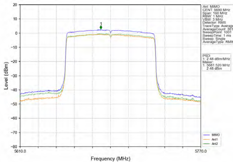
802.11ax(HEW80) HCH 5690MHz RU996 Left MIMO NTNv
