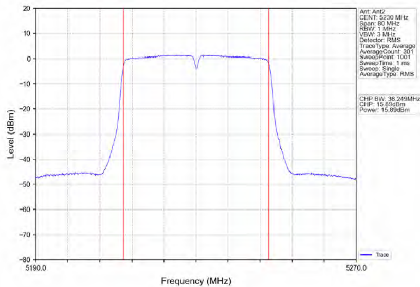
802.11n(HT40)_HCH_5230MHz_Ant2_NTN
