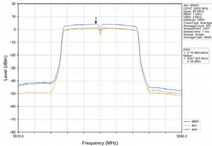
802.11n(HT40) MCH 5550MHz MIMO NTV
