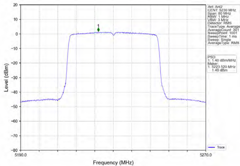
802.11ax(HEW40) HCH 5230MHz RU484 Left Ant2 NTNv
