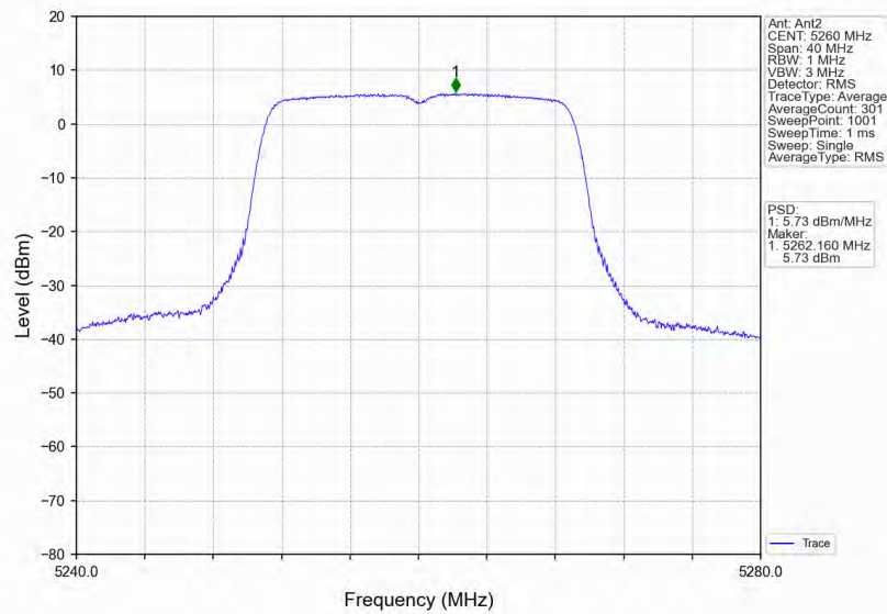
802.11n(HT20) LCH 5260MHz MIMO NTN
