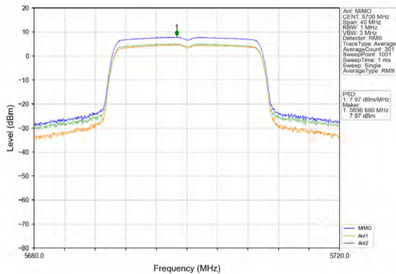
802.11ax(HEW20) HCH 5700MHz RU242 Left MIMO NTN
