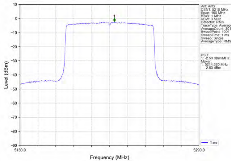
802.11ax(HEW80) MCH 5210MHz RU996 Left MIMO NTN
