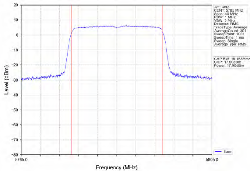
802.11ax(HEW20) MCH 5785MHz RU242 Left Ant2 NTNv
