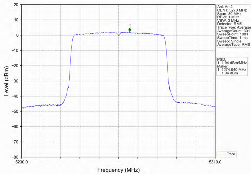
802.11ax(HEW40) LCH 5270MHz RU484 Left MIMO NTN
