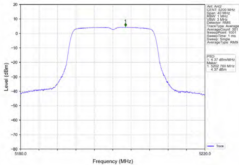
802.11n(HT20) MCH 5200MHz MIMO NTV
