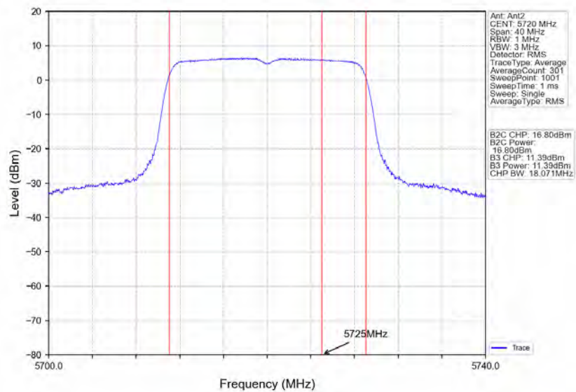
802.11n(HT20)_HCH_5720MHz_Ant2_NTN
