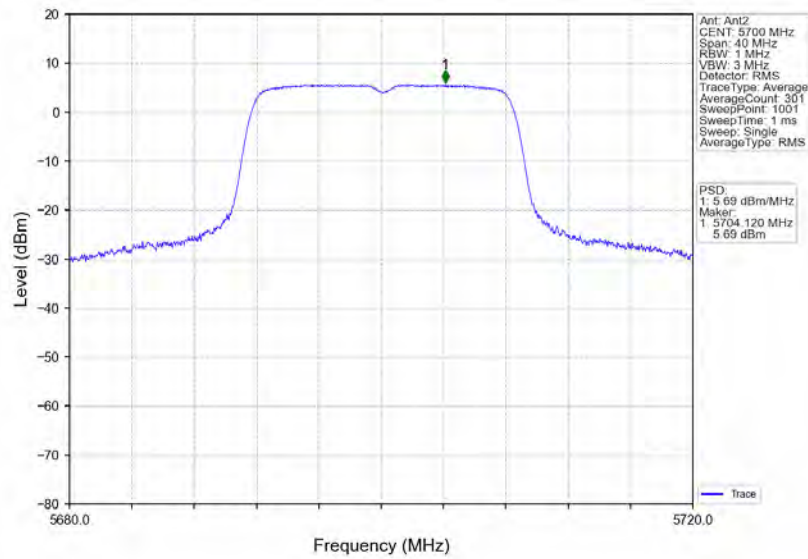
802.11a HCH 5700MHz Ant2 NTNv
