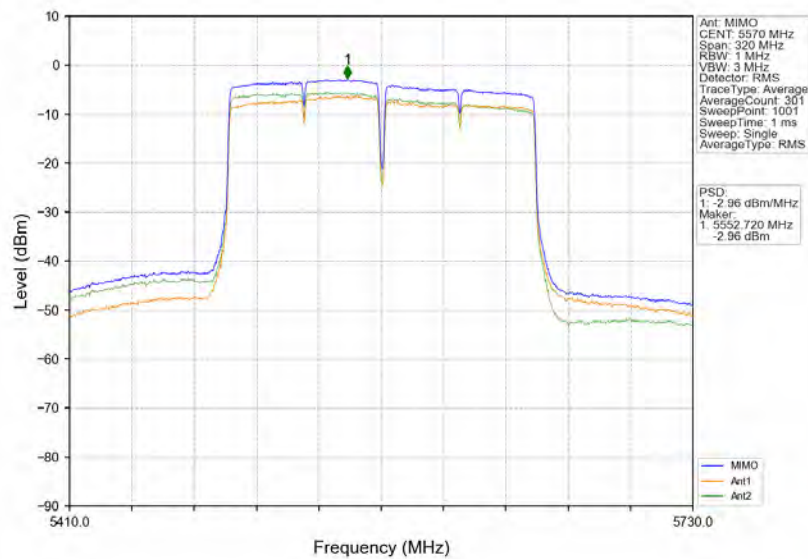
802.11ac(VHT160) MCH 5570MHz MIMO NTN
