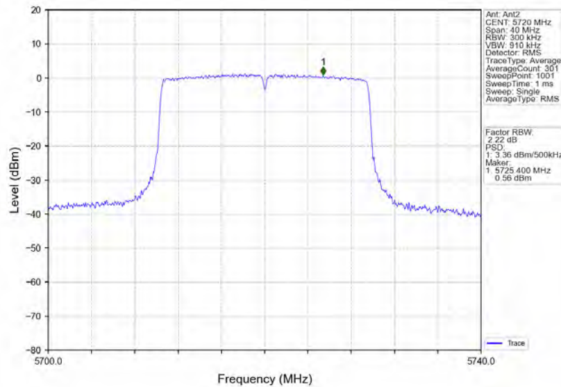
802.11ax(HEW20) HCH 5720MHz RU242 Left Ant2 NTNv
