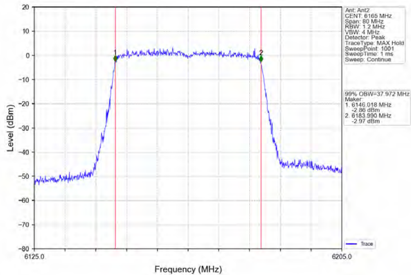
802.11ax(HEW40)_MCH_6165MHz_RU484_Left_Ant2_NTNV
