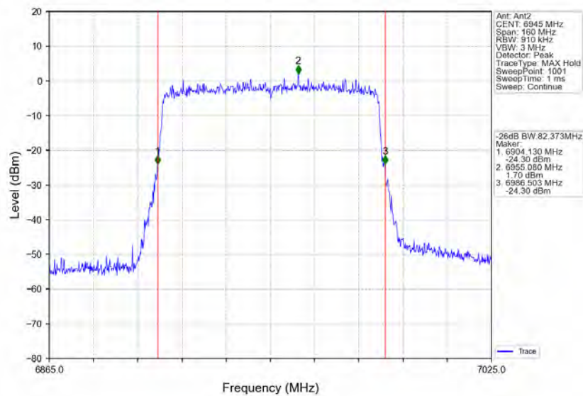
802.11ax(HEW80)_LCH_6945MHz_RU996_Left_Ant2_NTNV
