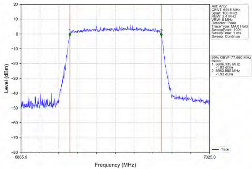
802.11ax(HEW80)_LCH_6945MHz_RU996_Left_Ant2_NTNV
