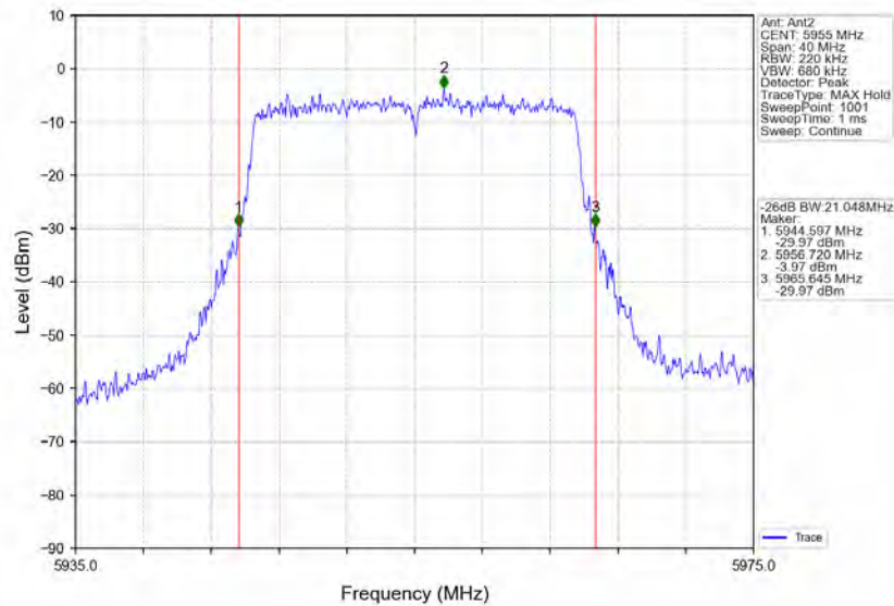
802.11ax(HEW20)_LCH_5955MHz_RU242_Left_Ant2_NTNV
