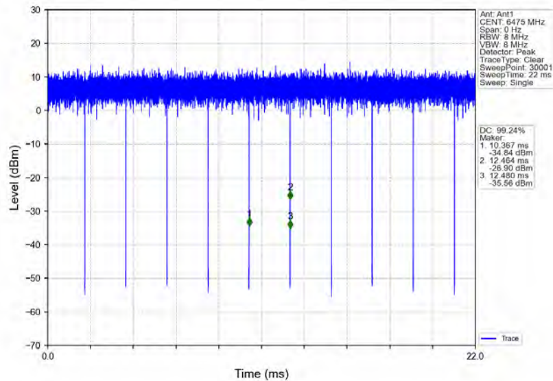
802.11a_MCH_6475MHz_Ant1_NTNV
