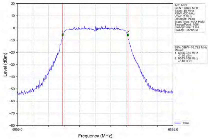
802.11a_HCH_6875MHz_Ant2_NTNV
