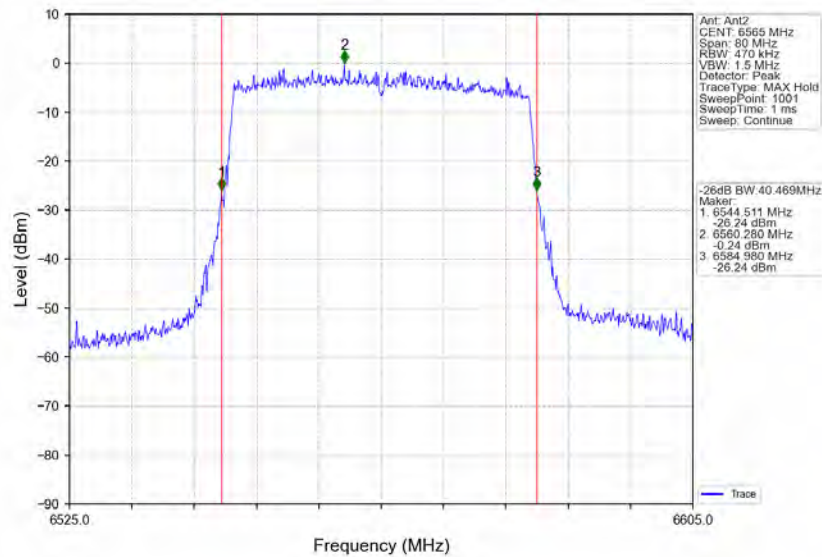
802.11ax(HEW40)_LCH_6565MHz_RU484_Left_Ant2_NTNV
