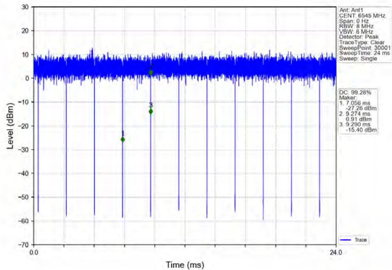
802.11ax(HEW80)_HCH_6545MHz_RU996_Left_Ant1_NTNV
