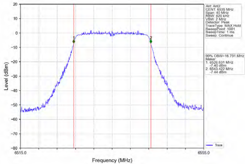
802.11a_LCH_6535MHz_Ant2_NTNV
