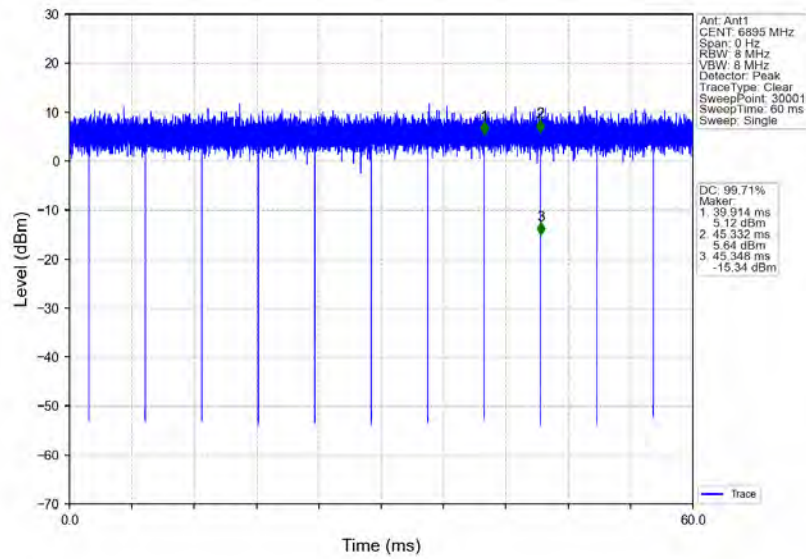
802.11ax(HEW20)_LCH_6895MHz_RU242_Left_Ant1_NTNV
