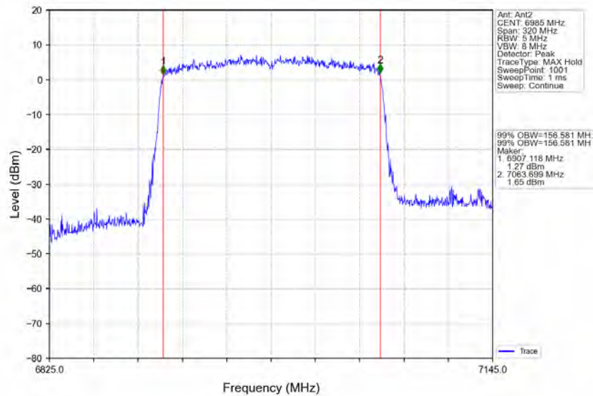
802.11ax(HEW160)_MCH_6985MHz_2xRU996_Left_Ant2_NTNV
