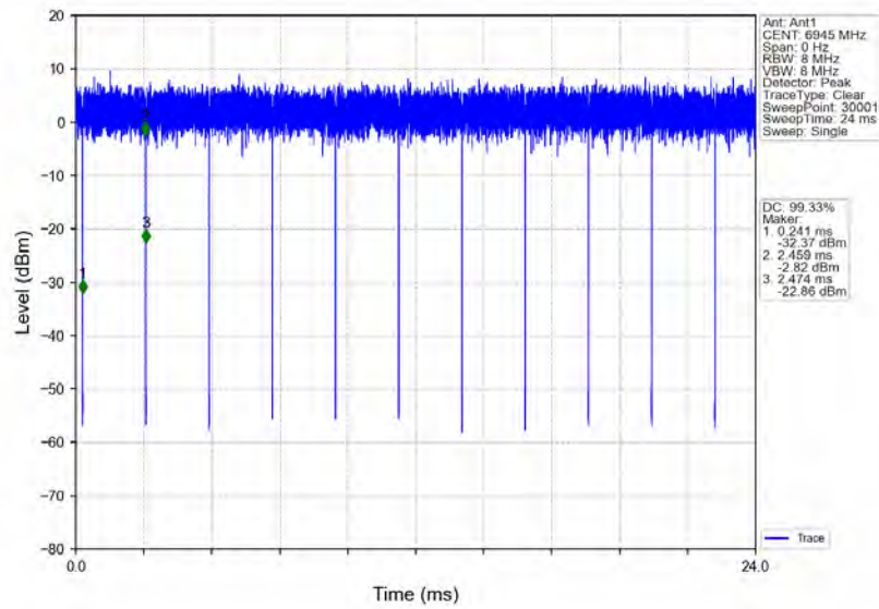
802.11ax(HEW80)_LCH_6945MHz_RU996_Left_Ant1_NTNV
