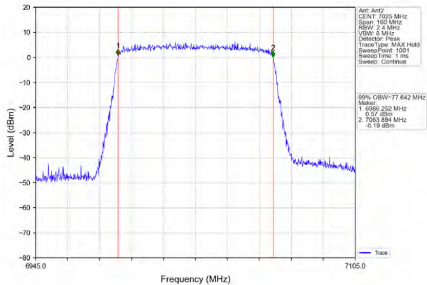
802.11ax(HEW80)_HCH_7025MHz_RU996_Left_Ant2_NTNV
