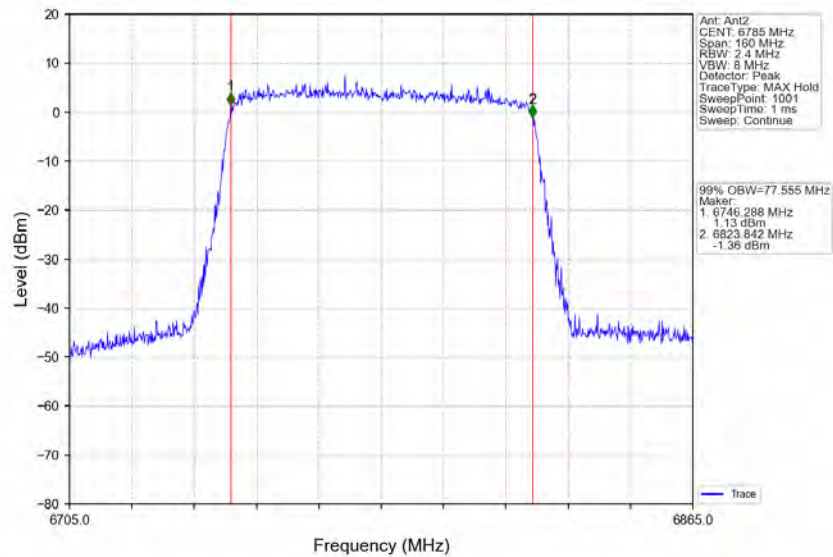
802.11ax(HEW80)_HCH_6785MHz_RU996_Left_Ant2_NTNV
