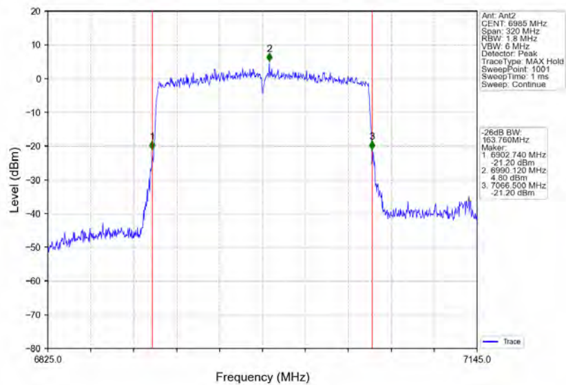
802.11ax(HEW160)_MCH_6985MHz_2xRU996_Left_Ant2_NTNV
