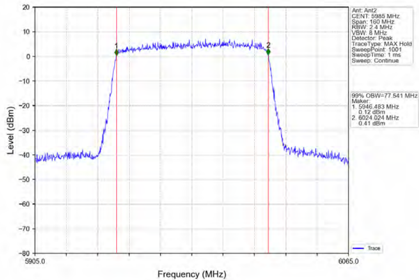
802.11ax(HEW80)_LCH_5985MHz_RU996_Left_Ant2_NTNV
