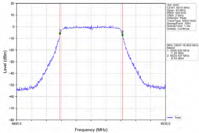
802.11a_HCH_6515MHz_Ant2_NTNV
