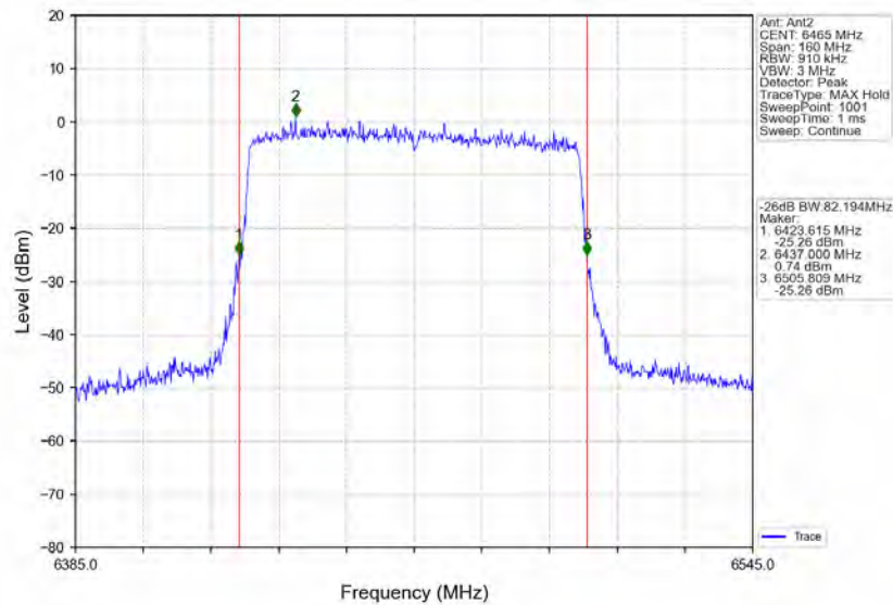
802.11ax(HEW80)_LCH_6465MHz_RU996_Left_Ant2_NTNV
