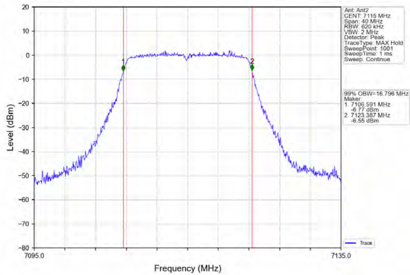
802.11a_HCH_7115MHz_Ant2_NTNV
