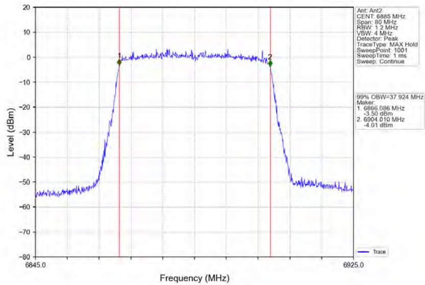
802.11ax(HEW40)_HCH_6885MHz_RU484_Left_Ant2_NTNV
