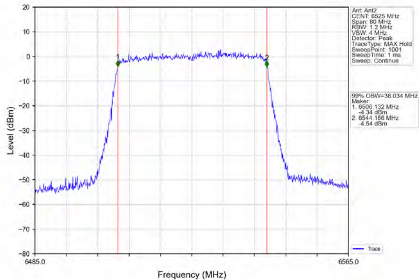
802.11ax(HEW40)_HCH_6525MHz_RU484_Left_Ant2_NTNV
