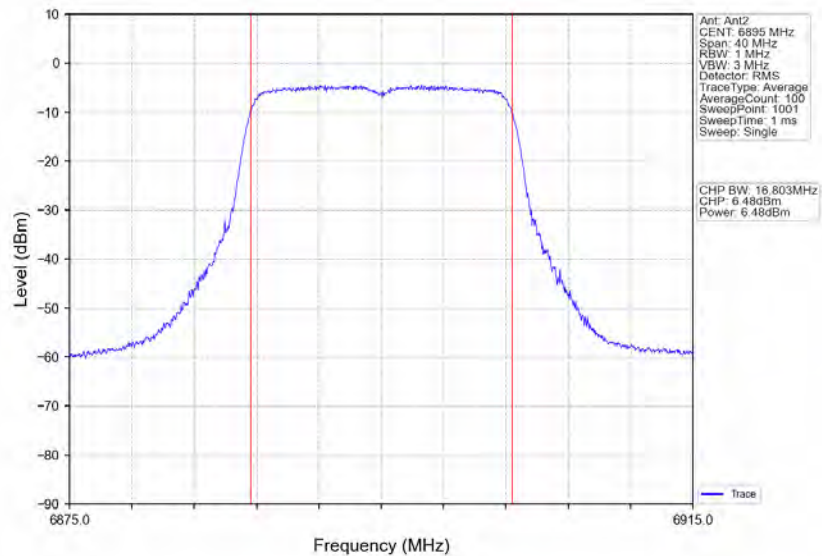
802.11a_LCH_6895MHz_Ant2_NTNV
