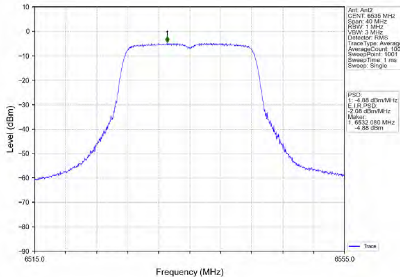
802.11a_LCH_6535MHz_Ant2_NTNV
