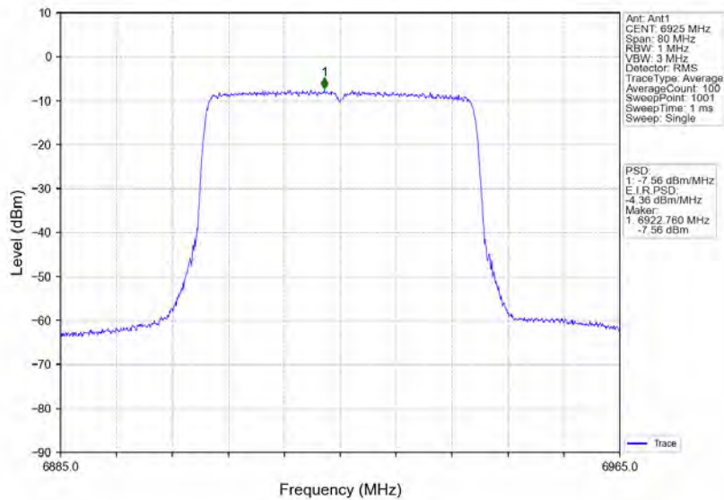
802.11ax(HEW40)_LCH_6925MHz_RU484_Left_Ant1_NTNV
