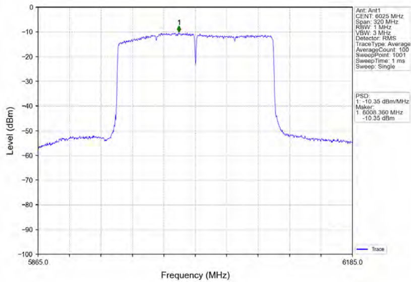
802.11ax(HEW160)_LCH_6025MHz_2xRU996_Left_Ant1_NTNV
