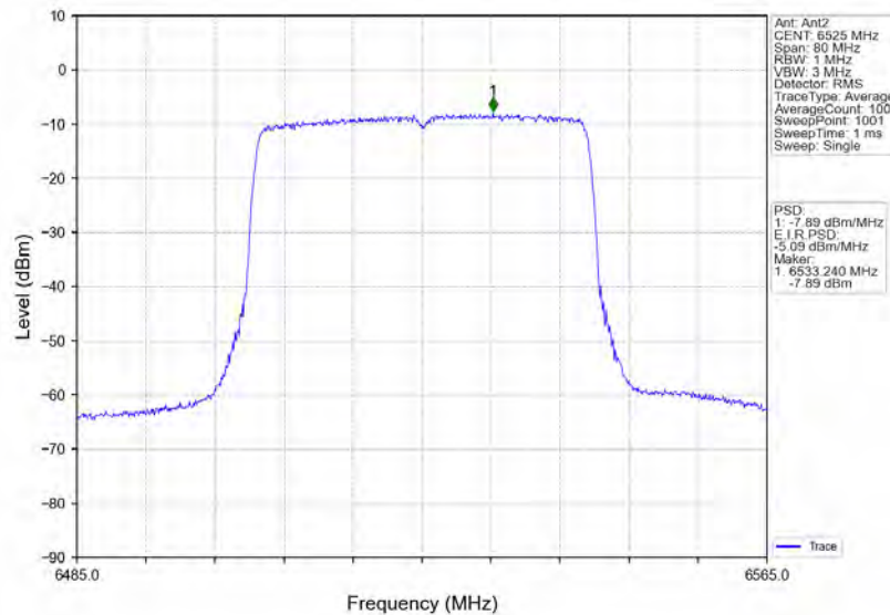
802.11ax(HEW40)_HCH_6525MHz_RU484_Left_Ant2_NTNV
