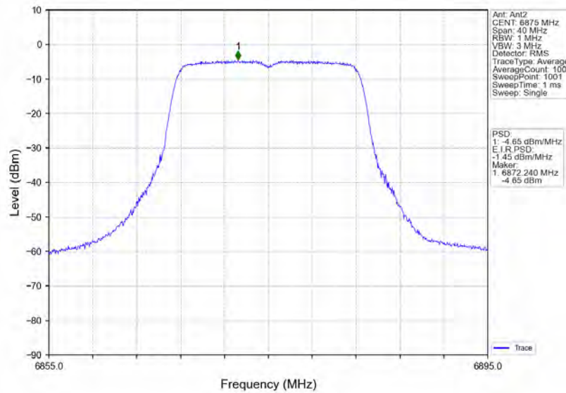
802.11a_HCH_6875MHz_Ant2_NTNV
