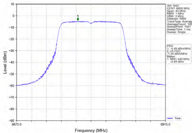
802.11a_LCH_6895MHz_Ant2_NTNV
