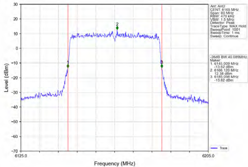
802.11ax(HEW40)_MCH_6165MHz_RU484_Left_Ant2_NTNV
