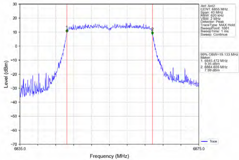
802.11ax(HEW20)_HCH_6855MHz_RU242_Left_Ant2_NTNV
