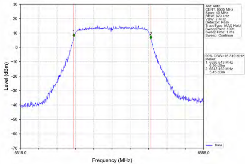
802.11a_LCH_6535MHz_Ant2_NTNV
