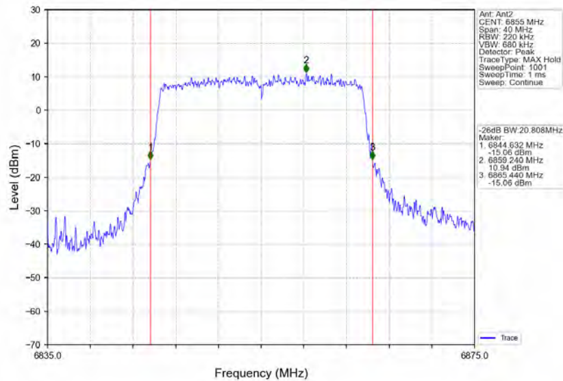
802.11ax(HEW20)_HCH_6855MHz_RU242_Left_Ant2_NTNV
