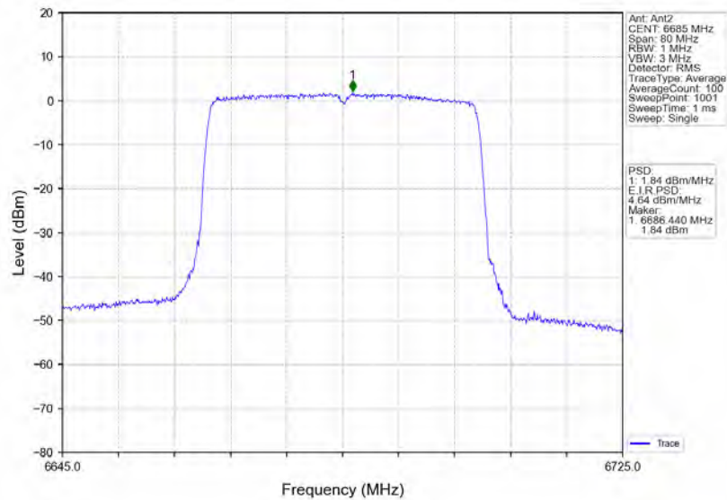
802.11ax(HEW40)_MCH_6685MHz_RU484_Left_Ant2_NTNV
