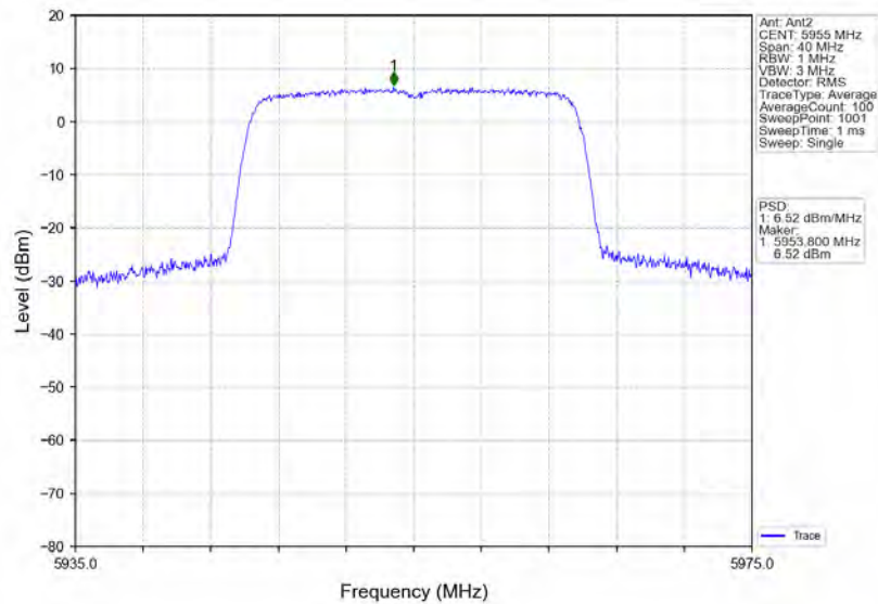
802.11ax(HEW20)_LCH_5955MHz_RU242_Left_Ant2_NTNV
