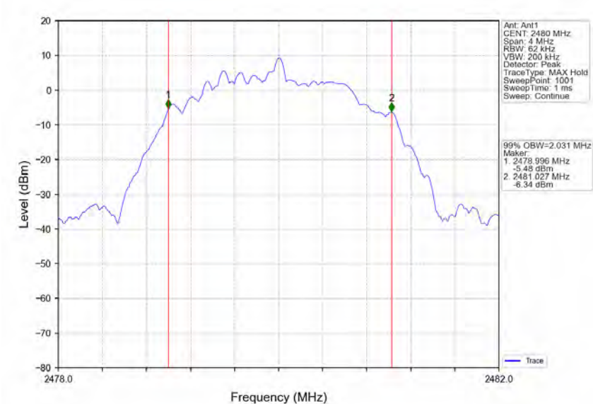
2M_HCH_2480MHz_Ant1_NTNV
