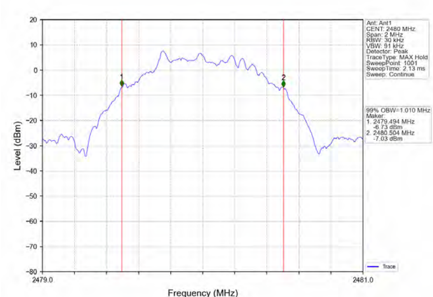
S2_HCH_2480MHz_Ant1_NTNV
