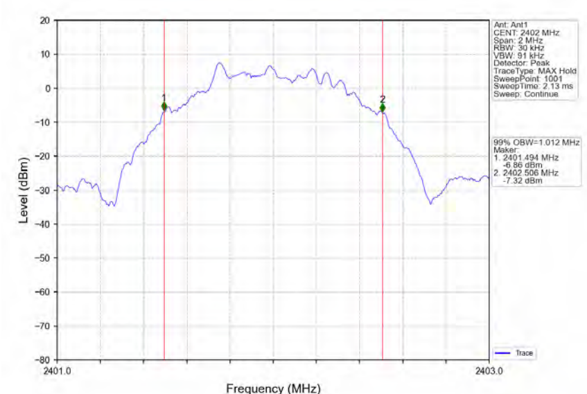
S2_LCH_2402MHz_Ant1_NTNV
