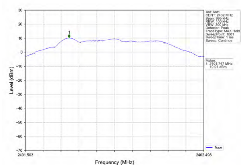
S2_LCH_2402MHz_Ant1_NTNV
