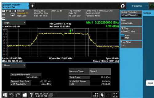
11N40MIMO-Ant0-5270
