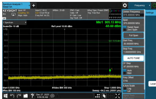
BLE_2M-Ant0-2440-30~1000-PASS
