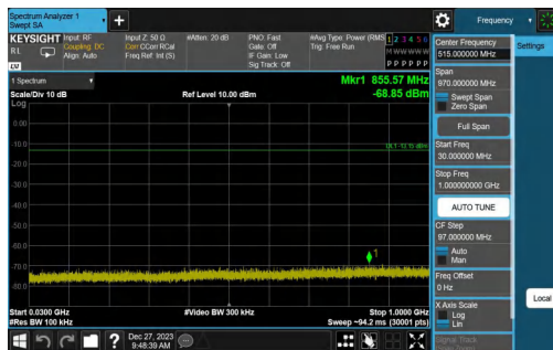
BLE_1M-Ant0-2440-30~1000-PASS
