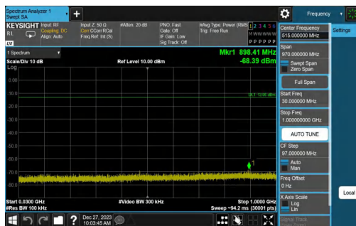
BLE_2M-Ant0-2480-30~1000-PASS
