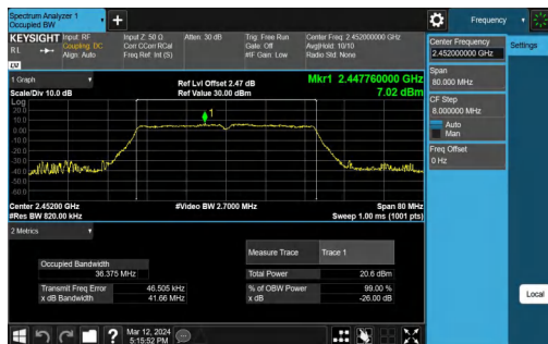
11N40MIMO-Ant0-2452
