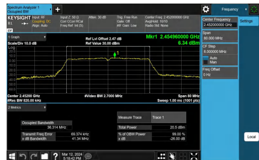
11N40MIMO-Ant1-2452
