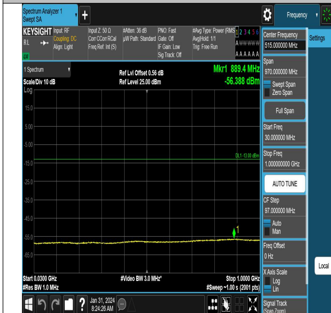
Band4-1312-30~1000MHz-PASS
