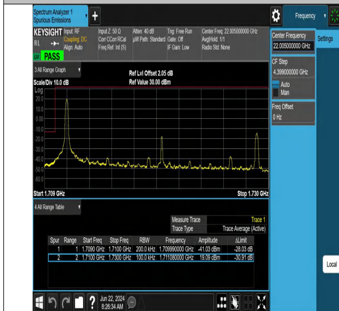
Band66-20MHz-QPSK-132072-1RB#0-PASS
