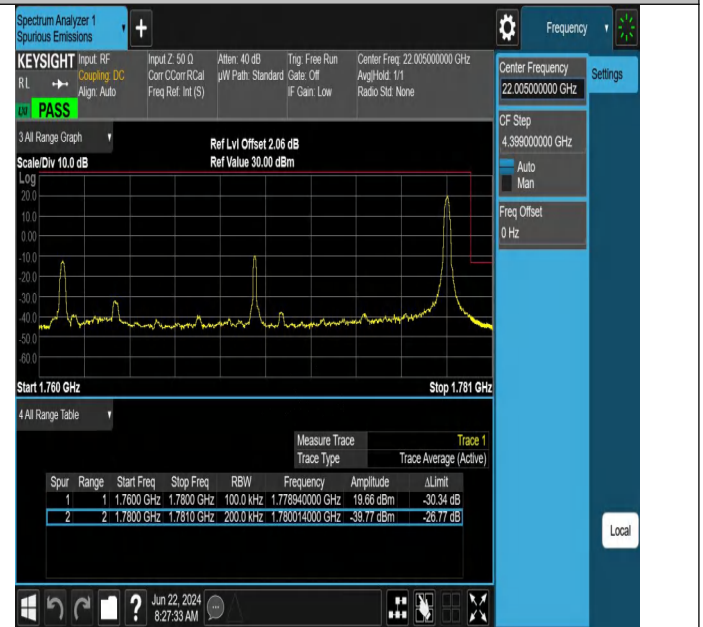
Band66-20MHz-QPSK-132572-1RB#99-PASS
