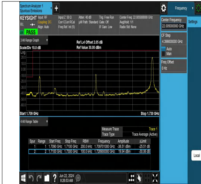
Band66-20MHz-QPSK-132072-1RB#99-PASS
