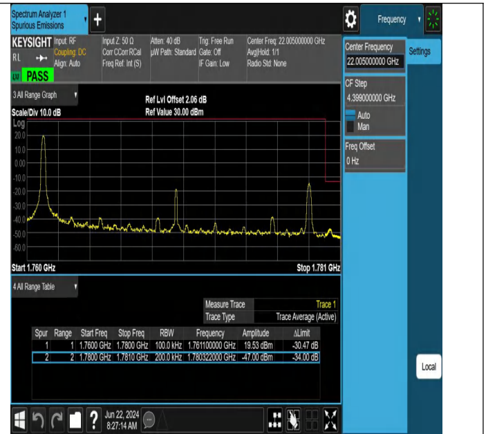
Band66-20MHz-QPSK-132572-1RB#0-PASS
