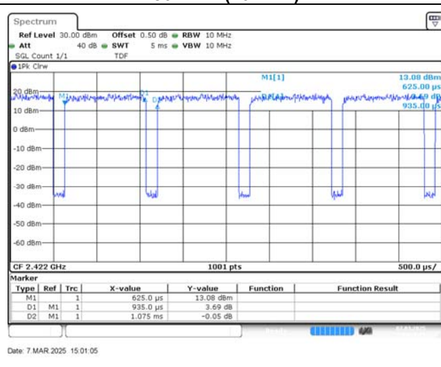
802.11n (40 MHz)
