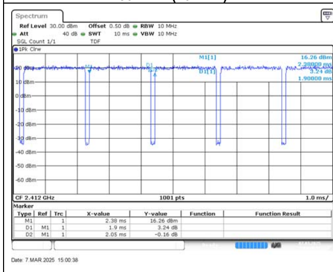
802.11n (20 MHz)
