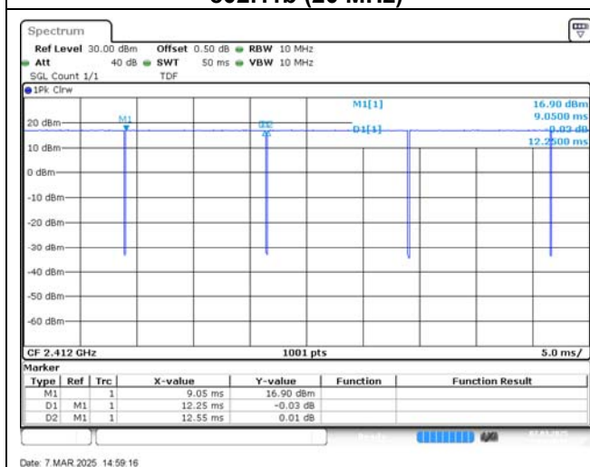
802.11b (20 MHz)
