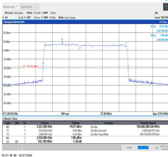
NTNV_CA_n41C_PC3_30+30_60+80_M+M_Ant1_TID9_1_#1
