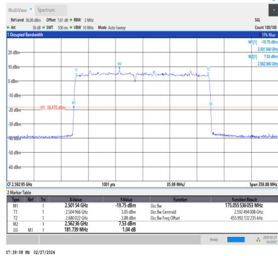
NTNV_CA_n41C_PC3_30+30_80+100_M+M_Ant1_TID7_1_#1
