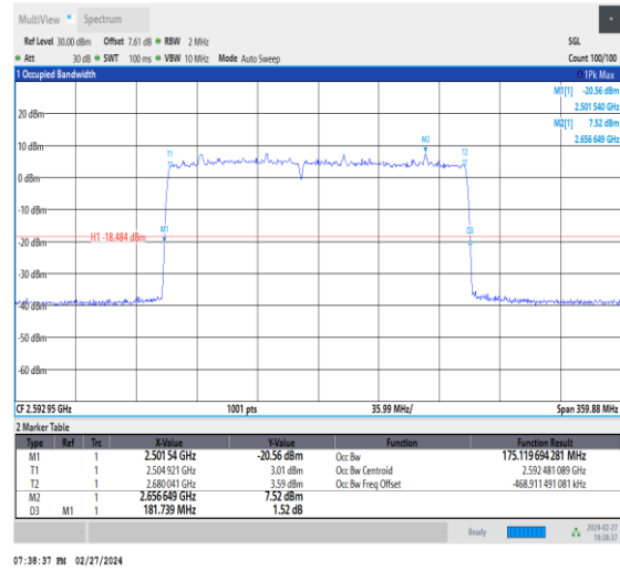
NTNV_CA_n41C_PC3_30+30_80+100_M+M_Ant1_TID5_1_#1
