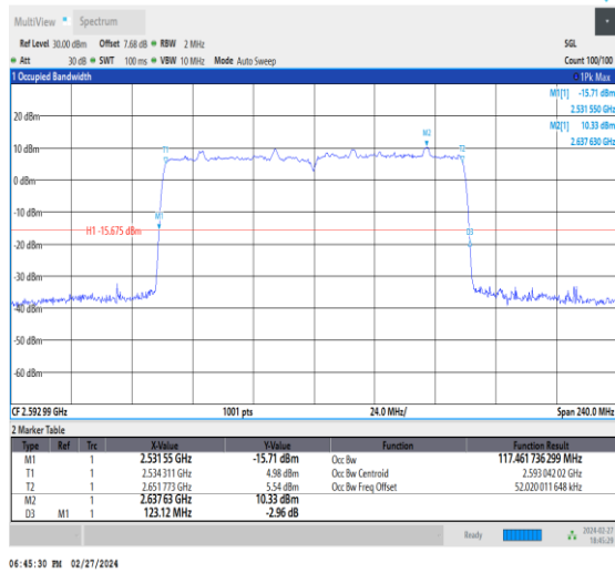
NTNV_CA_n41C_PC3_30+30_60+60_M+M_Ant1_TID8_1_#1
