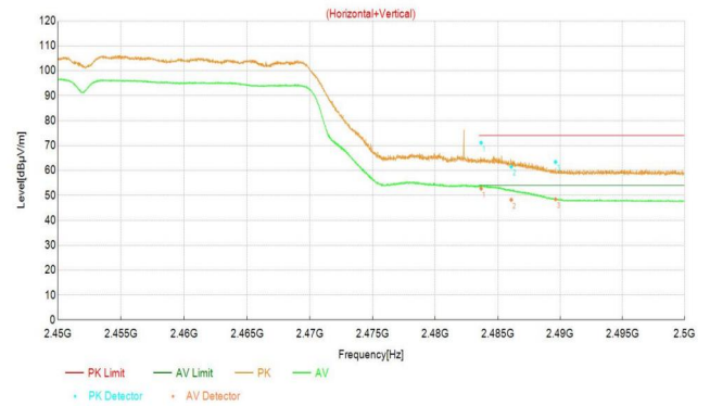
11n_40M_2452
