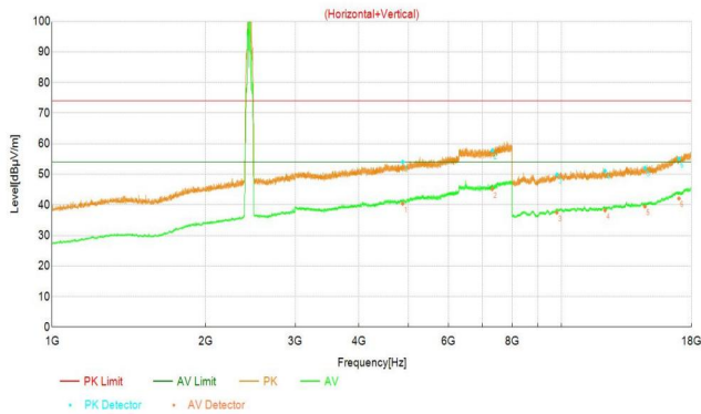
11n_40M_2437
