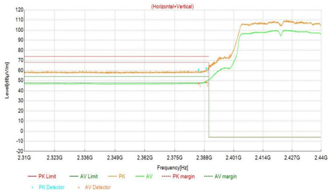
11n_40M_2422
