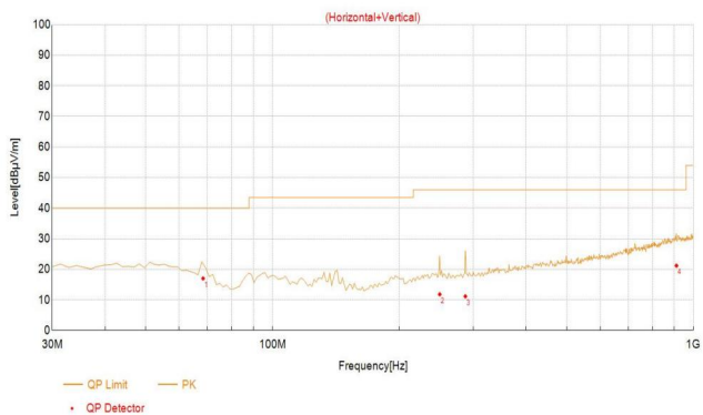
WIFI_2.4G_11b_20M_2462
