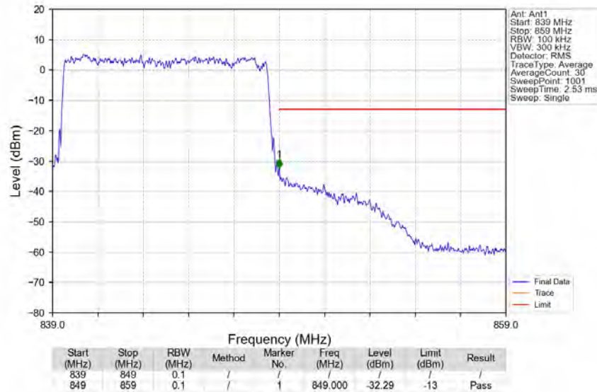
Band5_10MHz_QPSK_HCH_844MHz_RB_50_0_NTNV
