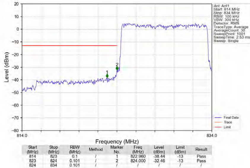
Band5_10MHz_QPSK_LCH_829MHz_RB_50_0_NTNV
