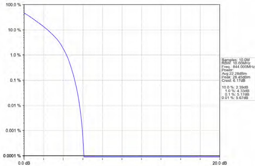
Band5_10MHz_QPSK_HCH_844MHz_RB_50_0_NTNV
