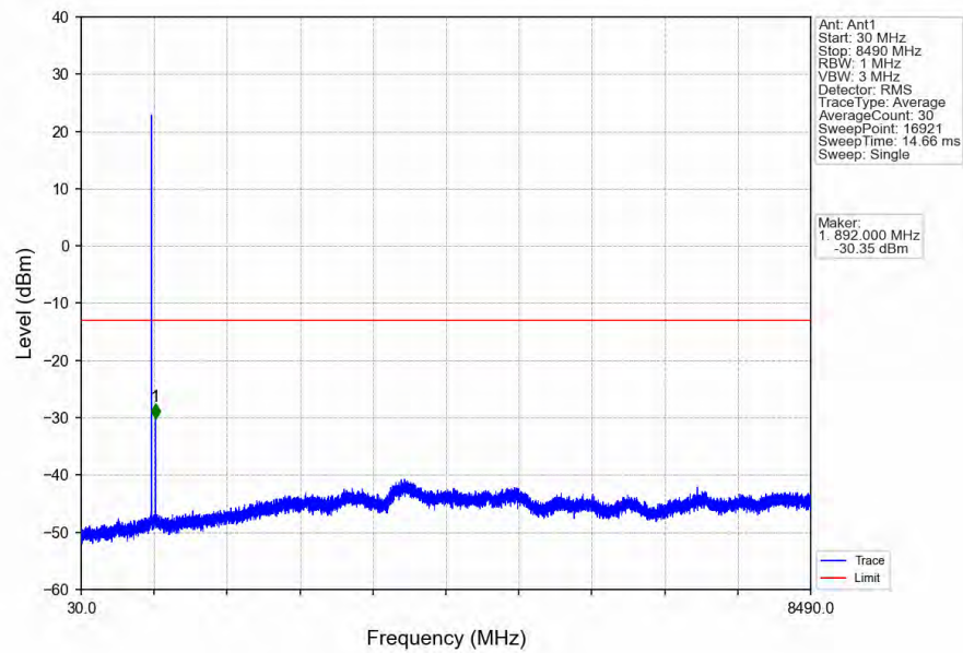
Band5_5MHz_QPSK_HCH_846.5MHz_RB_1_24_NTNV
