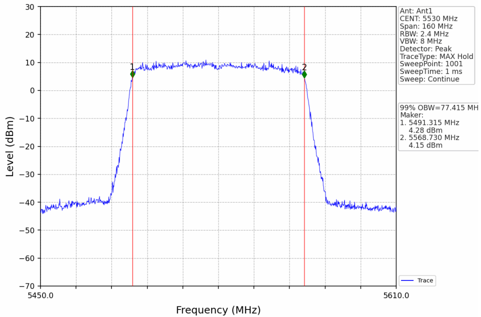
802.11ax(HE80)_LCH_5530MHz_RU996_Left_Ant1_NTNV
