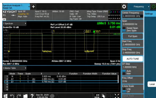
NTNV-DH5-Ant1-2480
