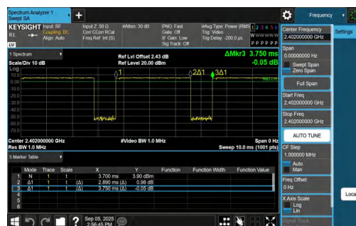
NTNV-2DH5-Ant1-2402
