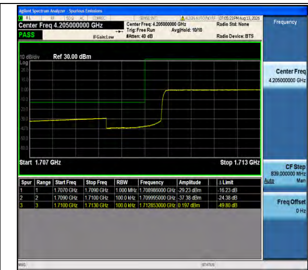
Band4-10MHz-QPSK-20000-50RB#0-PASS
