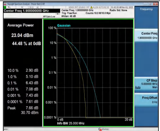
Band2-20MHz-16QAM-19100-27RB#0-PASS
