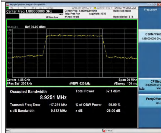
Band2-10MHz-QPSK-18900-50RB#0-PASS
