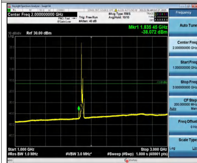
Band2-20MHz-QPSK-18900-1RB#0-1000~3000-PASS
