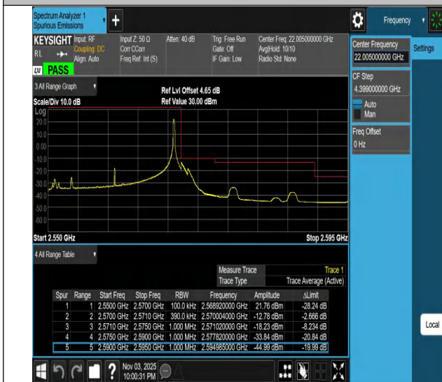
Band7-20MHz-QPSK-21350-1RB#99-PASS
