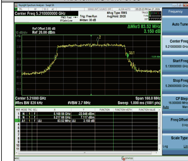
11be80MIMO-Ant1-5210
