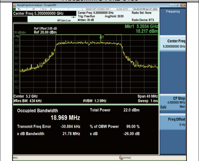
11be20MIMO-Ant2-5200
