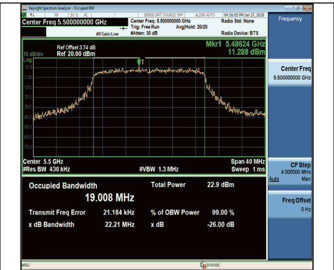
11be20MIMO-Ant2-5500
