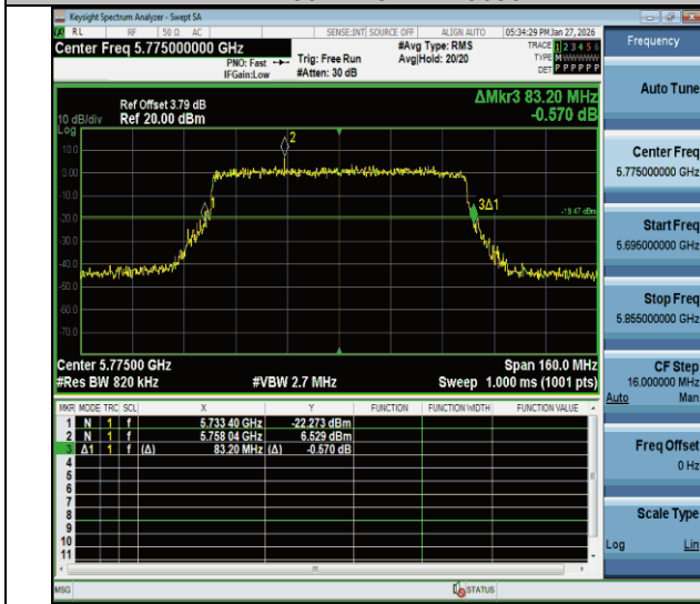
11be80MIMO-Ant1-5775
