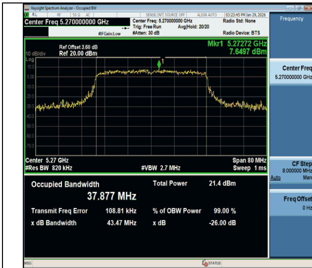
11be40MIMO-Ant1-5270
