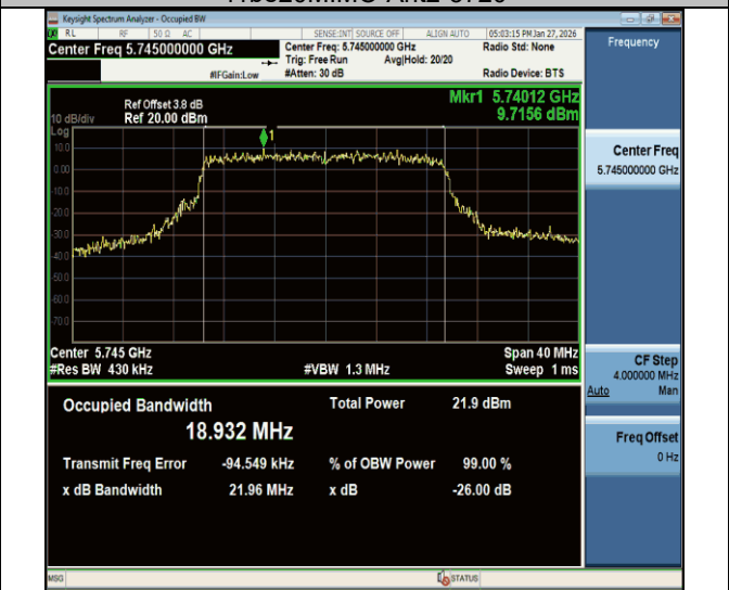
11be20MIMO-Ant2-5745
