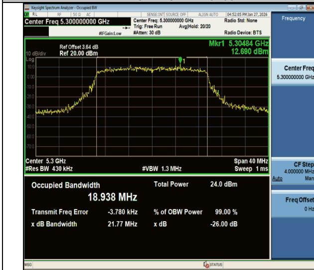
11be20MIMO-Ant1-5300
