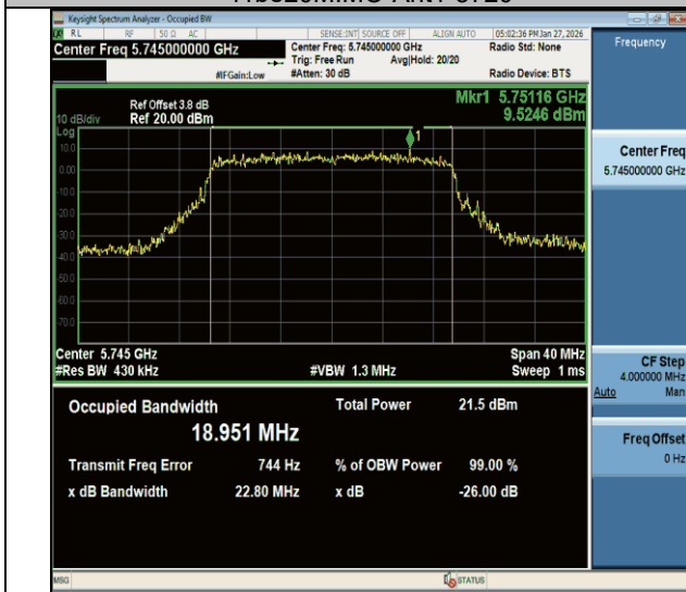
11be20MIMO-Ant1-5745
