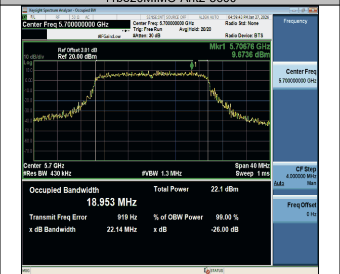
11be20MIMO-Ant2-5700
