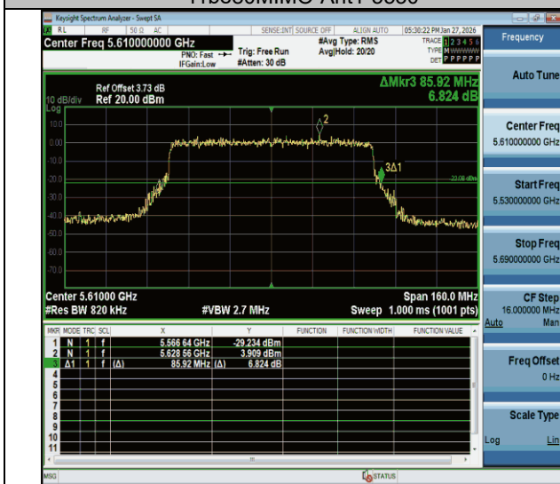
11be80MIMO-Ant1-5610
