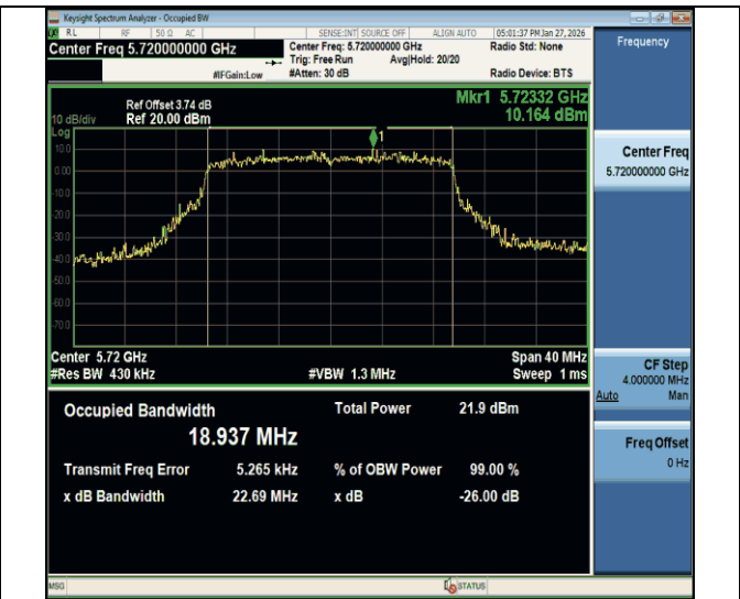
11be20MIMO-Ant2-5720
