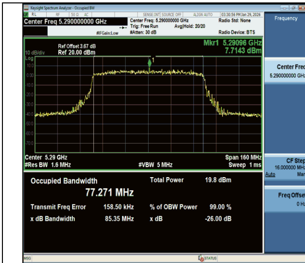
11be80MIMO-Ant1-5290
