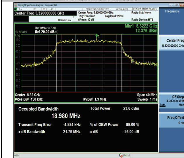
11be20MIMO-Ant1-5320
