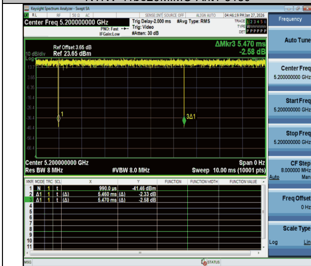
NTNV-11be20MIMO-Ant1-5200
