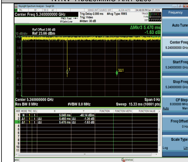
NTNV-11be20MIMO-Ant1-5240
