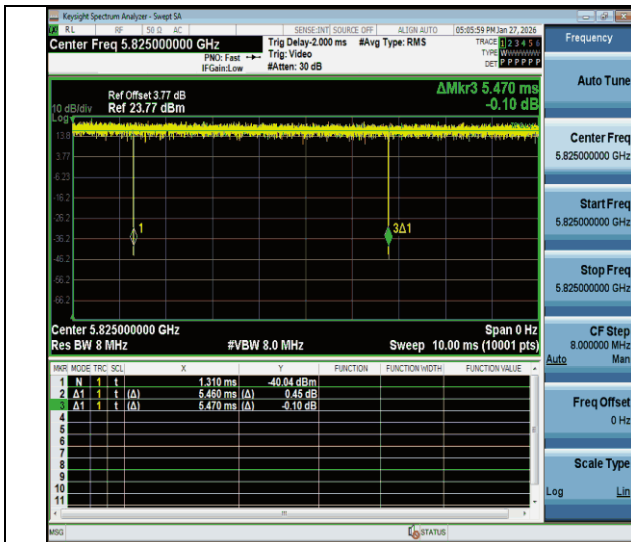
NTNV-11be20MIMO-Ant1-5825
