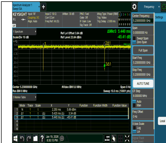
NTNV-11ac40MIMO-Ant1-5230
