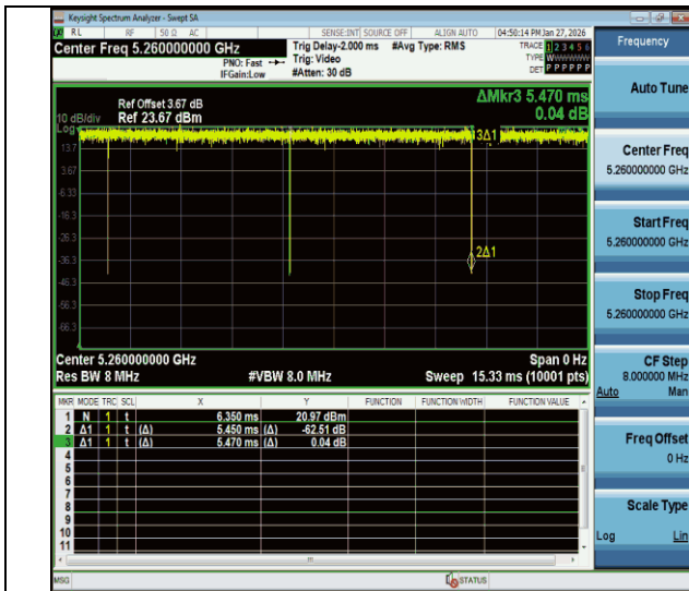
NTNV-11be20MIMO-Ant1-5260
