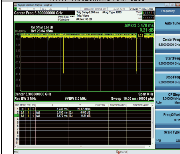
NTNV-11be20MIMO-Ant1-5300
