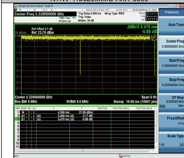
NTNV-11be20MIMO-Ant1-5320
