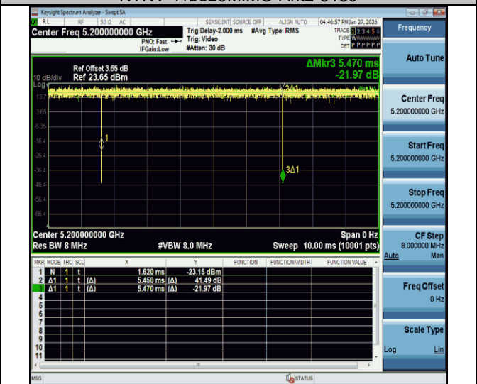
NTNV-11be20MIMO-Ant2-5200
