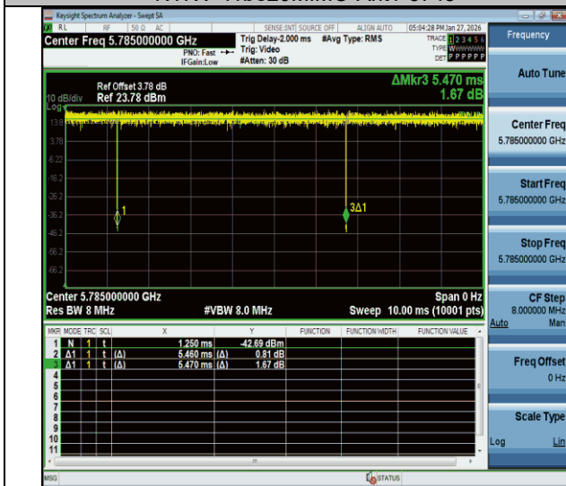
NTNV-11be20MIMO-Ant1-5785
