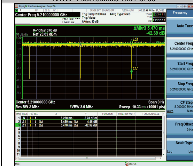
NTNV-11be80MIMO-Ant1-5210
