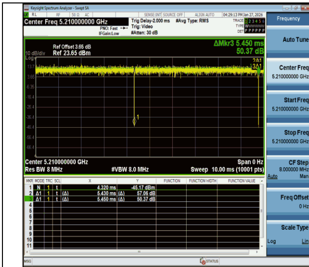
NTNV-11ac80MIMO-Ant1-5210
