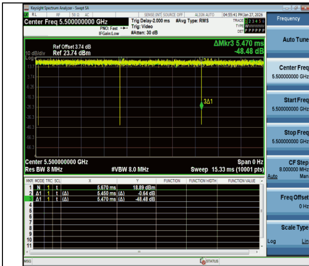
NTNV-11be20MIMO-Ant1-5500
