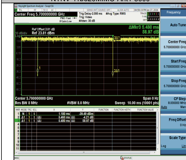
NTNV-11be20MIMO-Ant1-5700
