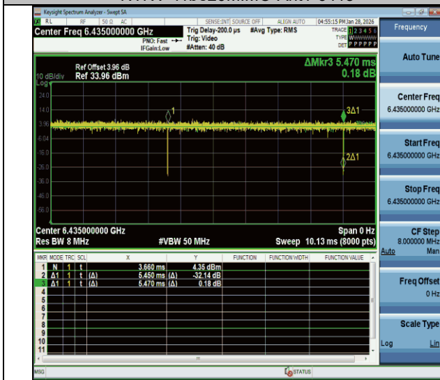
NTNV-11be20MIMO-Ant1-6435
