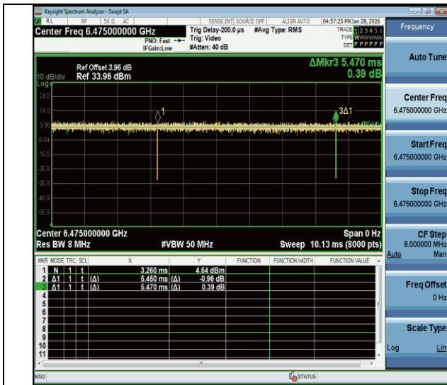
NTNV-11be20MIMO-Ant1-6475
