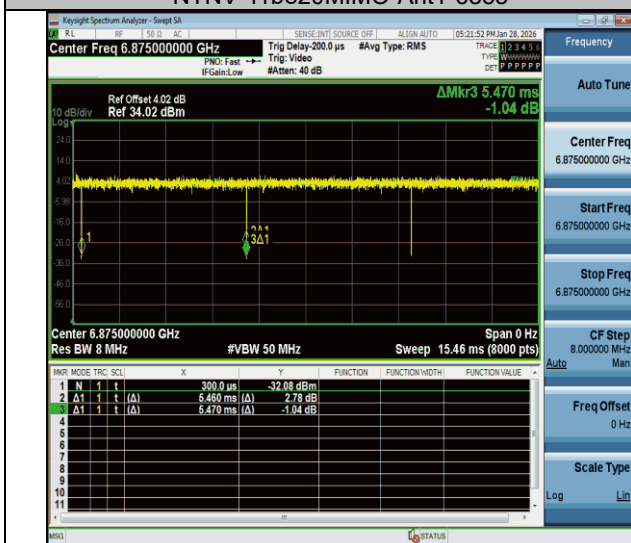
NTNV-11be20MIMO-Ant1-6875
