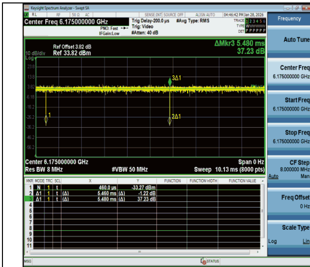
NTNV-11be20MIMO-Ant1-6175
