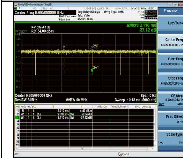
NTNV-11a-CDD-Ant1-6695
