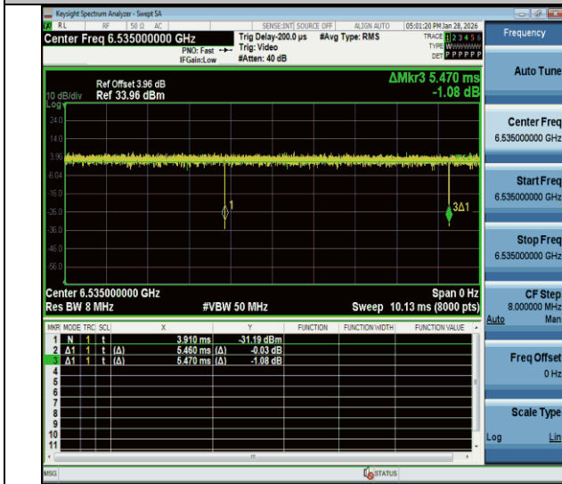
NTNV-11be20MIMO-Ant1-6535
