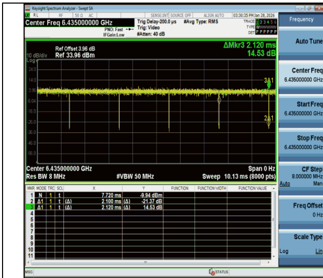
NTVN-11a-CDD-Ant1-6435
