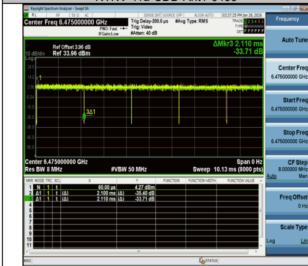
NTVN-11a-CDD-Ant1-6475
