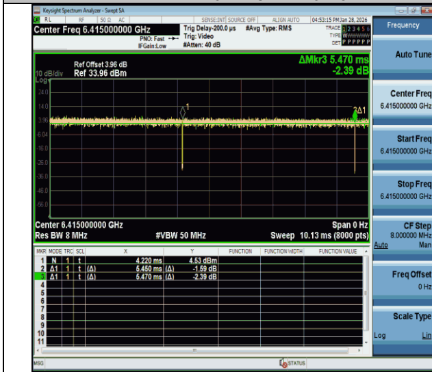
NTNV-11be20MIMO-Ant1-6415
