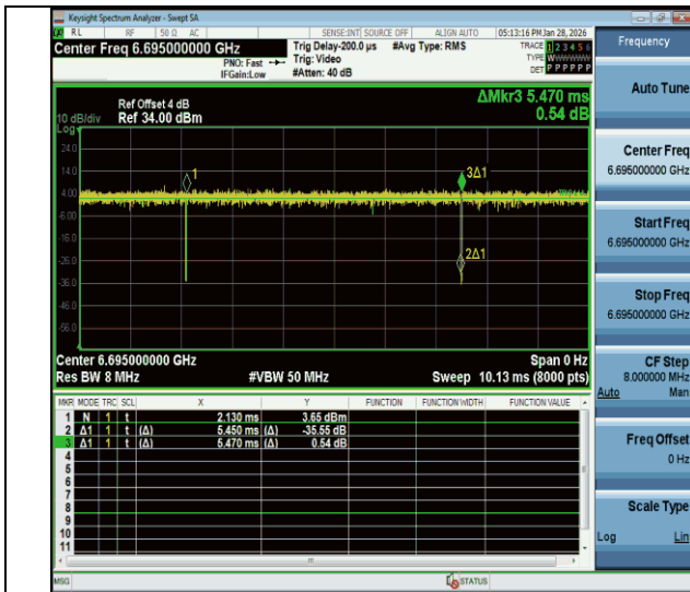
NTNV-11be20MIMO-Ant1-6695
