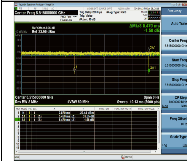
NTNV-11be20MIMO-Ant1-6515
