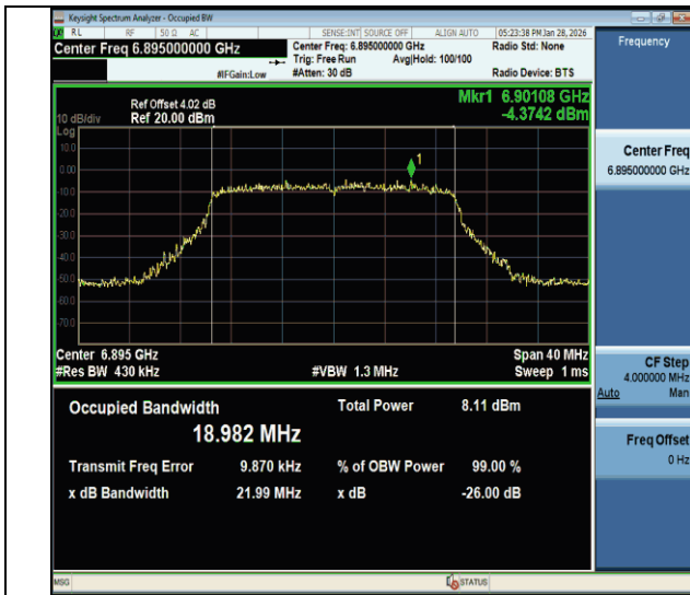
11be20MIMO-Ant1-6895-PASS
