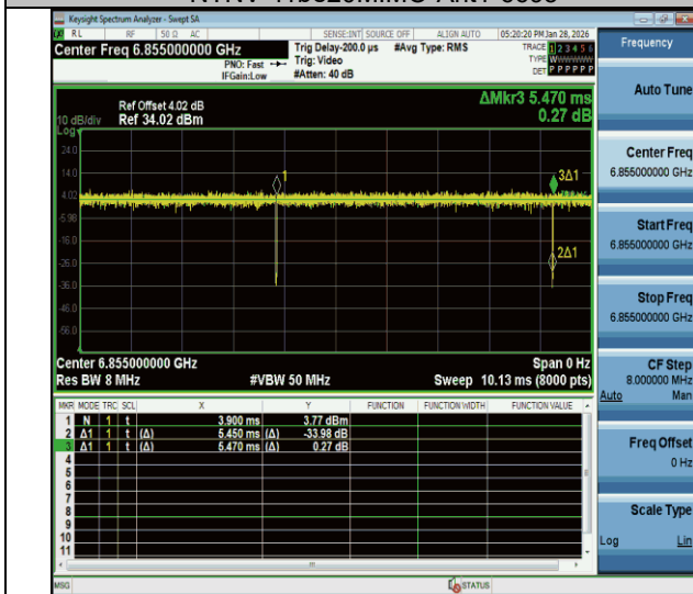
NTNV-11be20MIMO-Ant1-6855
