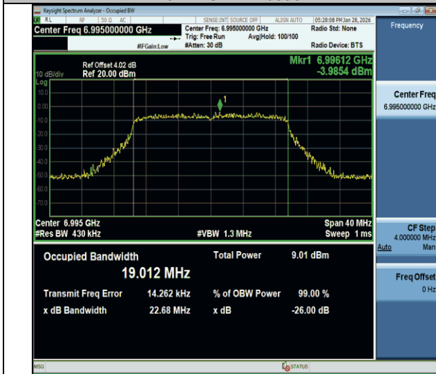
11be20MIMO-Ant1-6995-PASS
