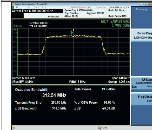
11be320MIMO-Ant1-6105-PASS
