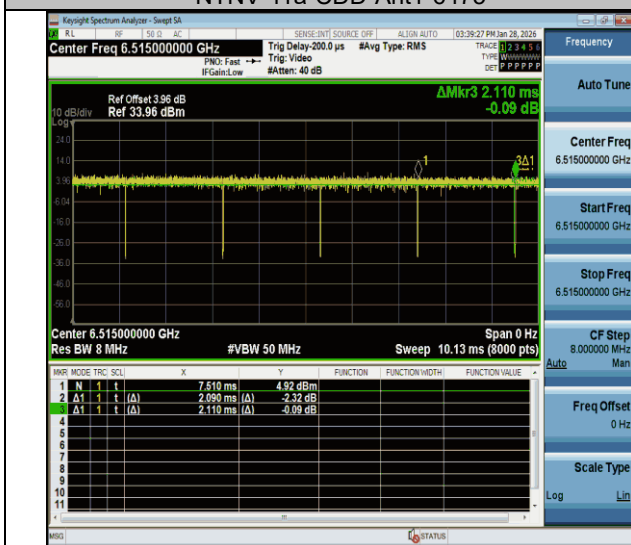
NTVN-11a-CDD-Ant1-6515
