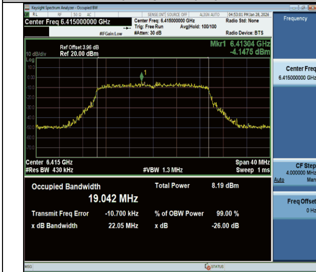
11be20MIMO-Ant1-6415-PASS
