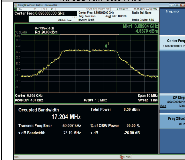
11a-CDD-Ant1-6695-PASS
