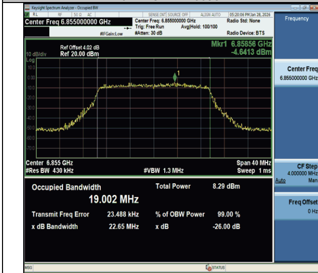
11be20MIMO-Ant1-6855-PASS
