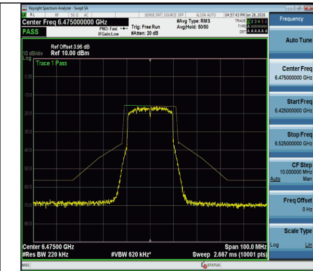
NTVN-11be20MIMO-Ant1-6475-PASS
