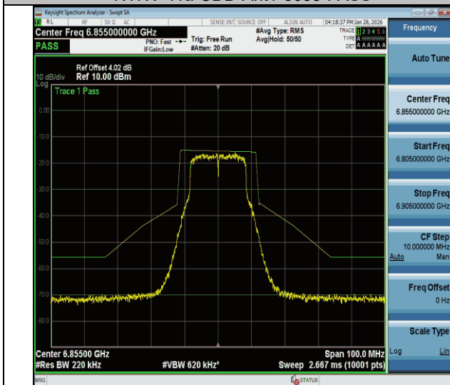
NTVN-11a-CDD-Ant1-6855-PASS
