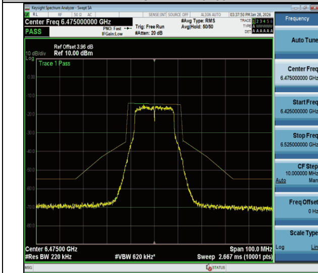
NTVN-11a-CDD-Ant1-6475-PASS
