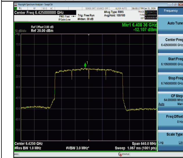
11be320MIMO-Ant1-6425-PASS
