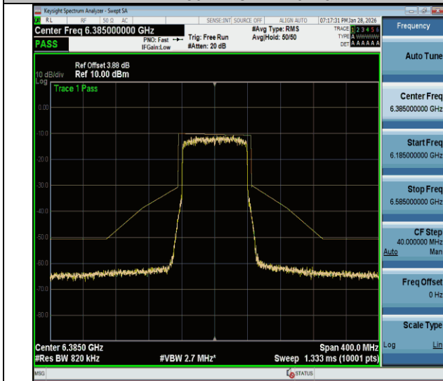
NTVN-11be80MIMO-Ant1-6385-PASS
