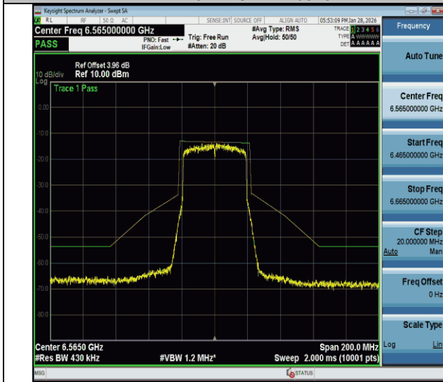
NTVN-11be40MIMO-Ant1-6565-PASS
