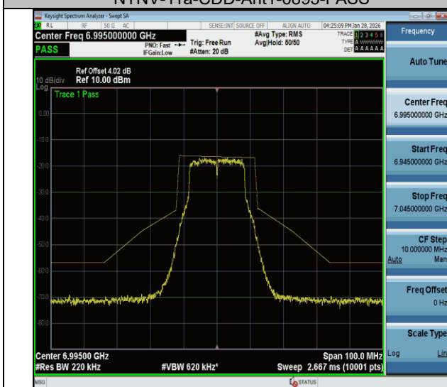
NTVN-11a-CDD-Ant1-6995-PASS
