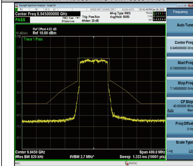
NTVN-11be80MIMO-Ant1-6945-PASS
