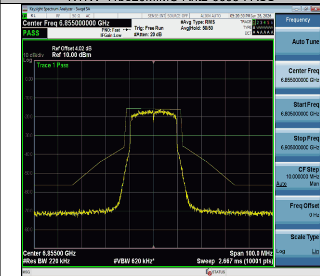
NTVN-11be20MIMO-Ant1-6855-PASS
