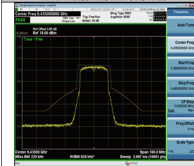
NTVN-11be20MIMO-Ant1-6435-PASS
