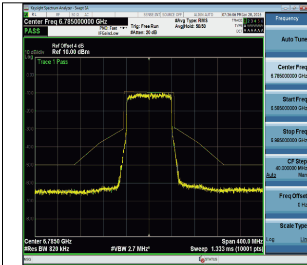
NTVN-11be80MIMO-Ant1-6785-PASS
