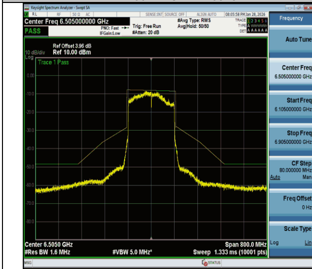
NTNV-11be160MIMO-Ant1-6505-PASS
