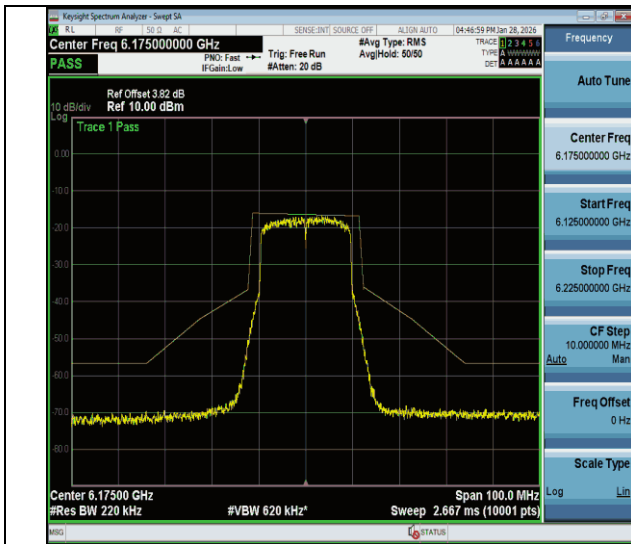
NTVN-11be20MIMO-Ant1-6175-PASS
