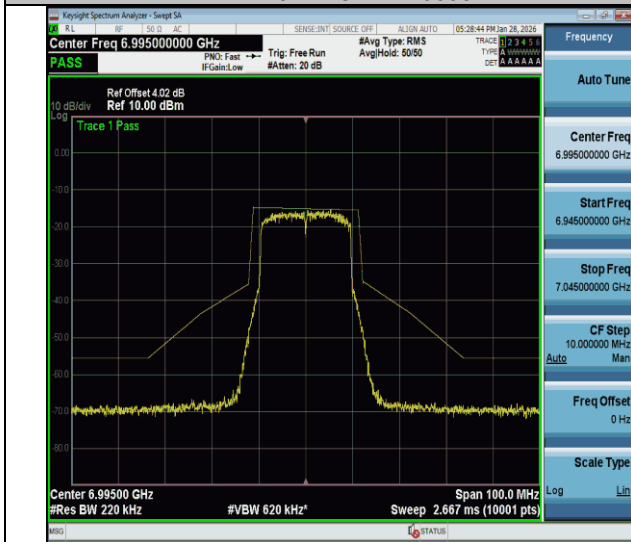
NTVN-11be20MIMO-Ant1-6995-PASS
