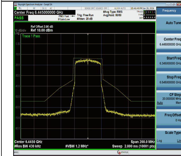
NTVN-11be40MIMO-Ant1-6445-PASS
