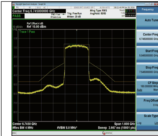
NTNV-11be320MIMO-Ant1-6745-PASS
