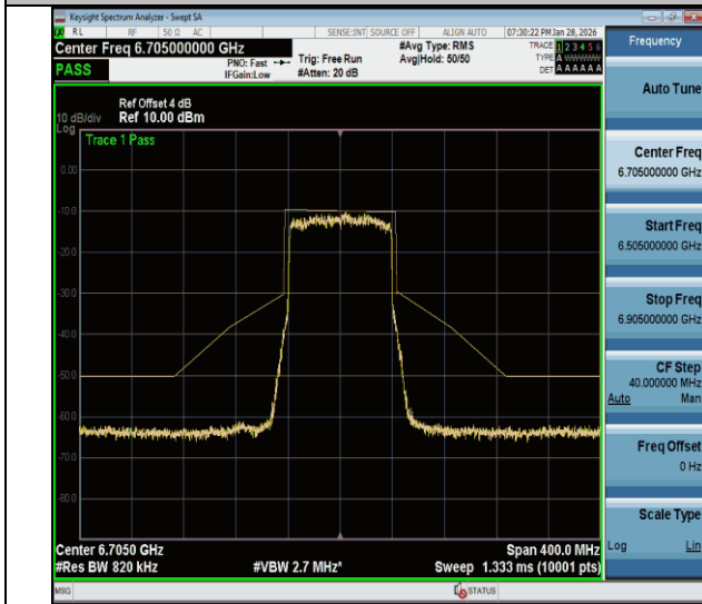
NTVN-11be80MIMO-Ant1-6705-PASS
