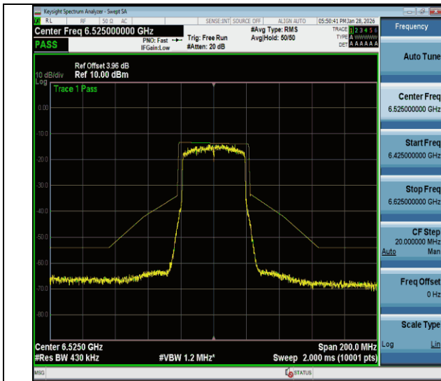
NTVN-11be40MIMO-Ant1-6525-PASS
