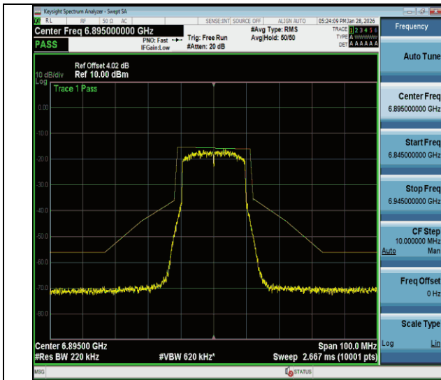
NTVN-11be20MIMO-Ant1-6895-PASS
