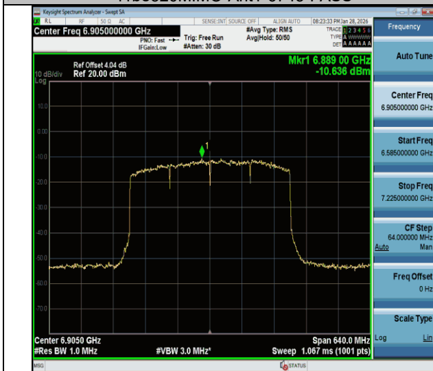
11be320MIMO-Ant1-6905-PASS
