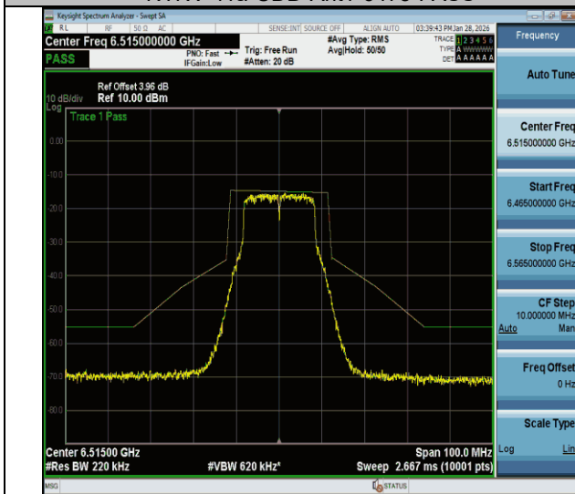
NTVN-11a-CDD-Ant1-6515-PASS
