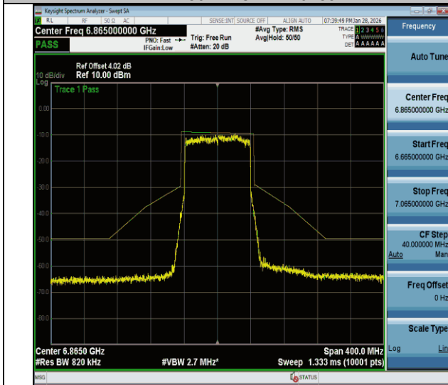
NTVN-11be80MIMO-Ant1-6865-PASS
