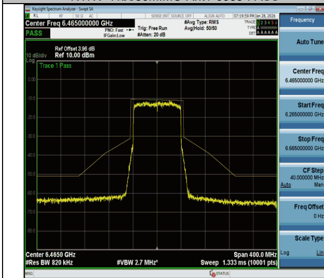
NTVN-11be80MIMO-Ant1-6465-PASS
