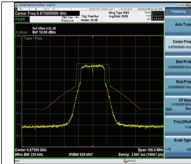
NTVN-11a-CDD-Ant1-6875-PASS
