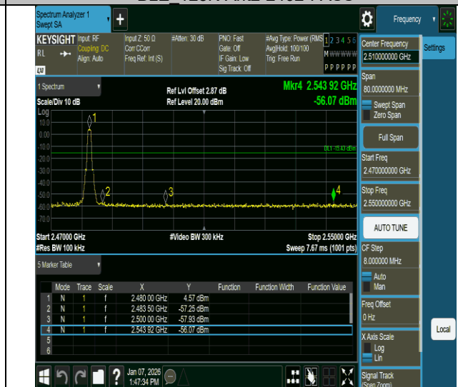
BLE 125K-Ant2-2480-PASS
