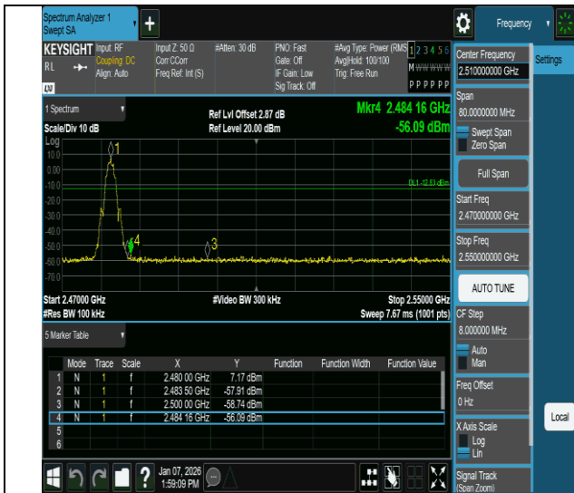
BLE 2M-Ant1-2480-PASS
