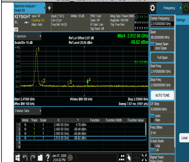
BLE 125K-Ant1-2480-PASS
