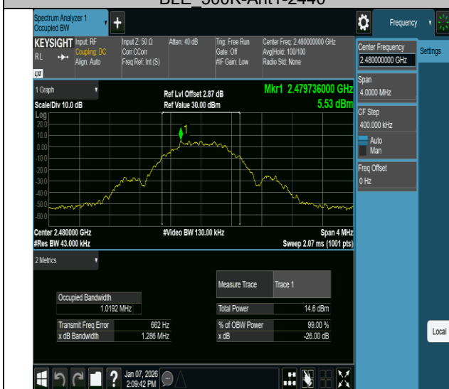
BLE_500K-Ant1-2480
