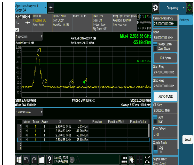
BLE 2M-Ant2-2480-PASS
