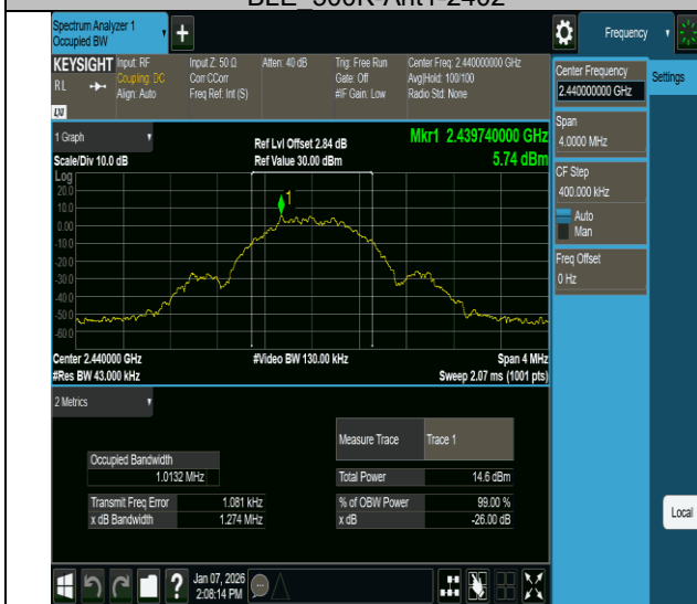
BLE_500K-Ant1-2440
