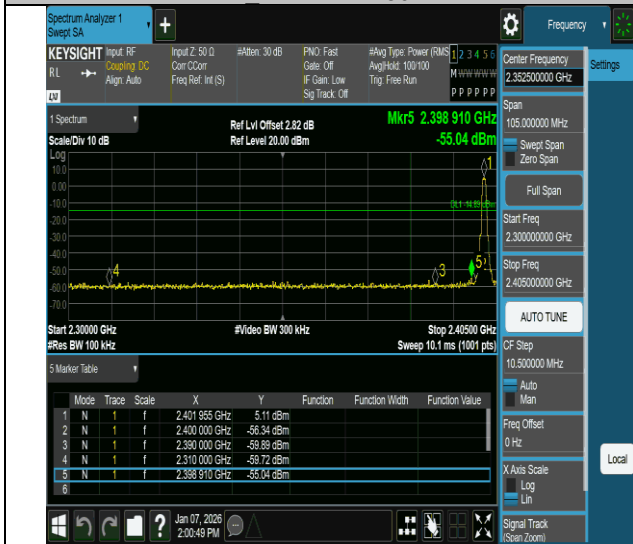
BLE 125K-Ant1-2402-PASS
