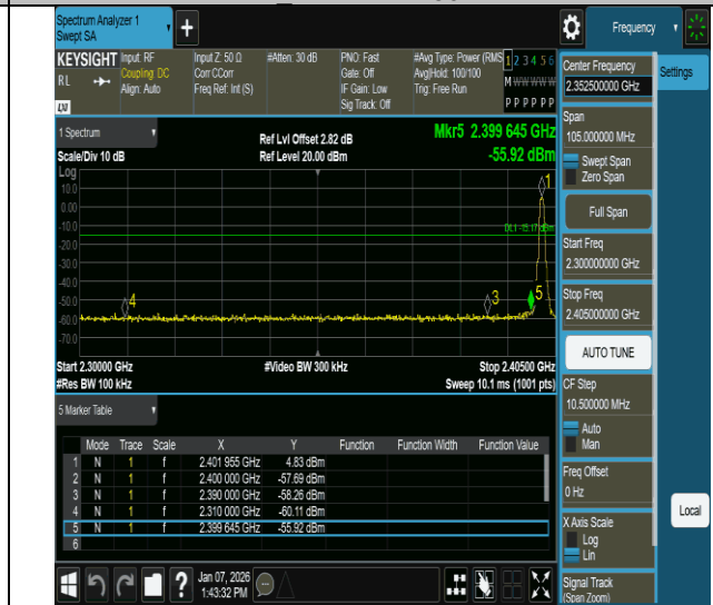
BLE 125K-Ant2-2402-PASS
