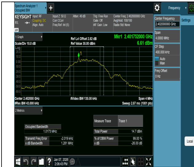
BLE_500K-Ant1-2402
