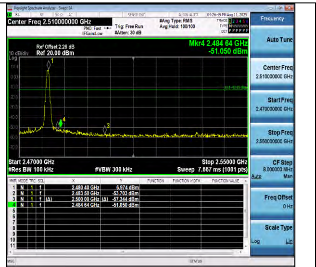
BLE 500K-Ant1-2480-PASS
