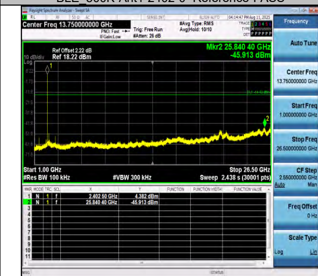
BLE 500K-Ant1-2402-1000~26500-PASS
