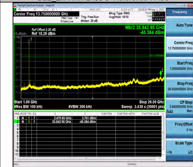
BLE 2M-Ant1-2480-1000~26500-PASS
