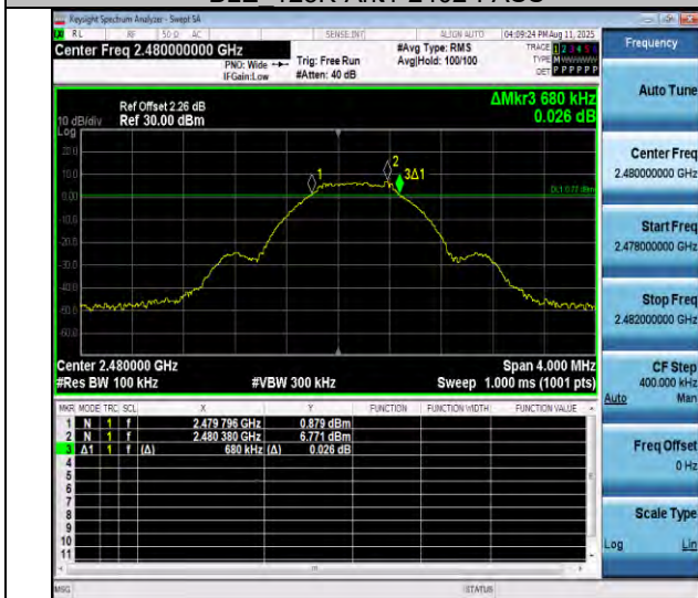
BLE 125K-Ant1-2480-PASS
