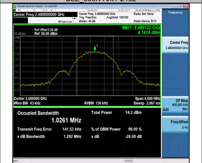
BLE 500K-Ant1-2480
