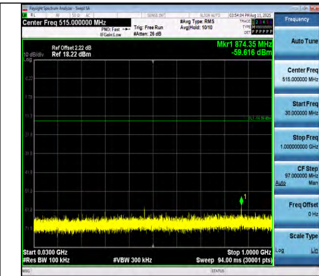
BLE 125K-Ant1-2402-30~1000-PASS
