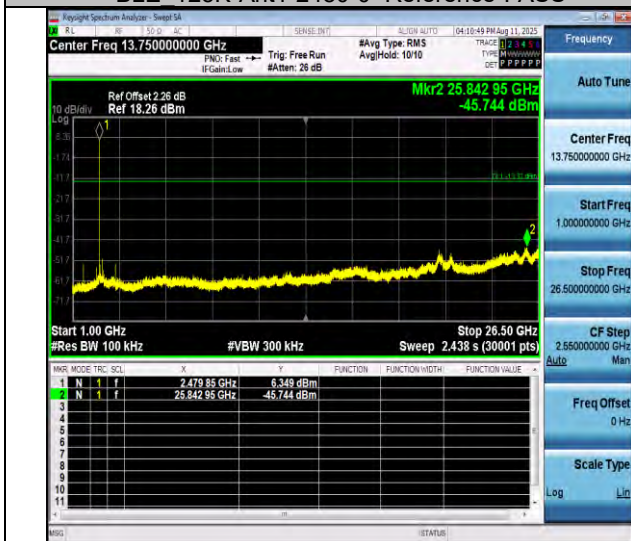
BLE 125K-Ant1-2480-1000~26500-PASS
