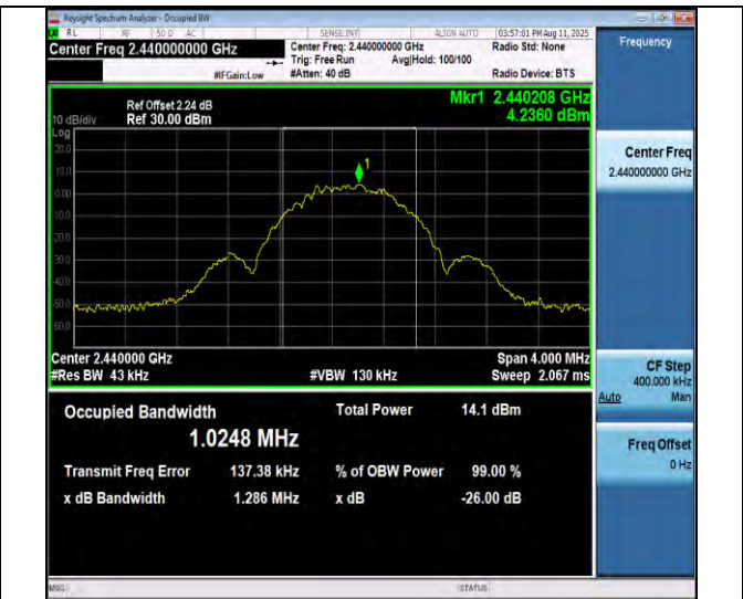
BLE 125K-Ant1-2440
