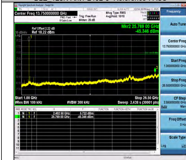
BLE 125K-Ant1-2402-1000~26500-PASS
